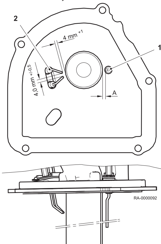
Obr.42 Elektrody
