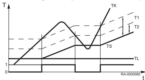
Obr.36 Regulace napouštění /schematická)
