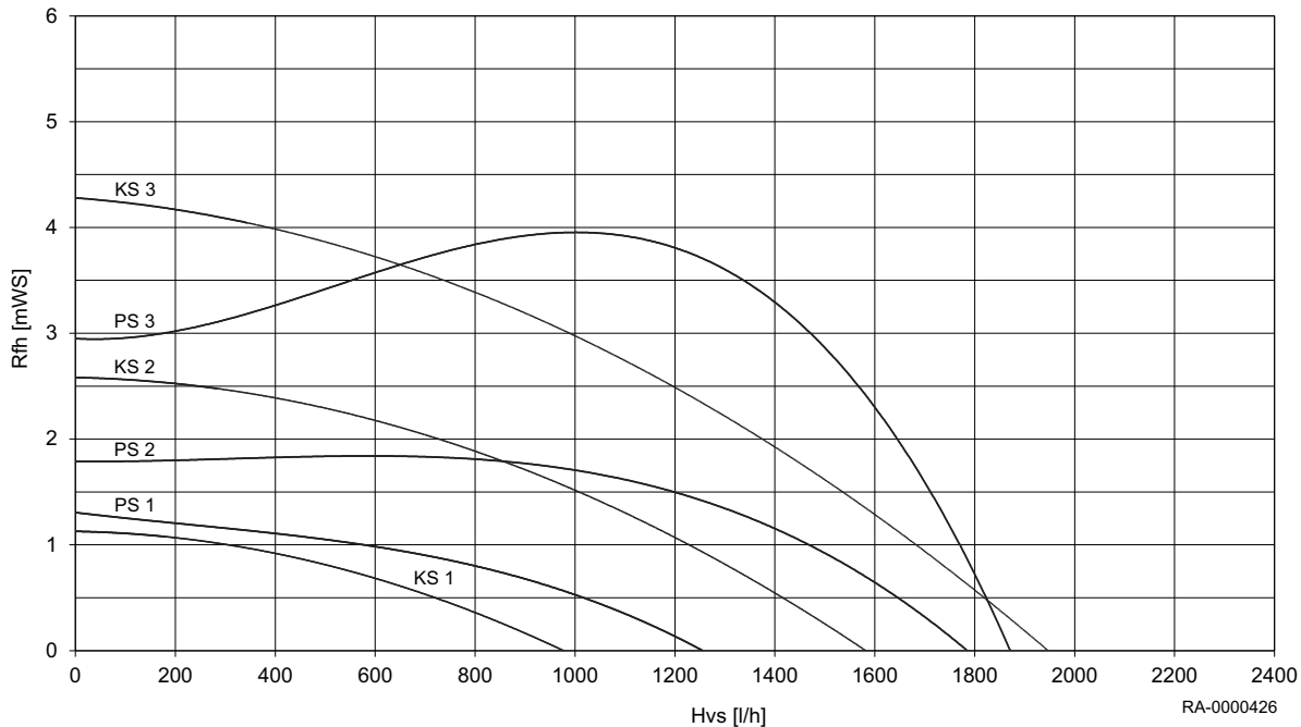
Obr.3 Celková dopravní výška WGB-M EVO pro mísicí topný okruh (úměrný či konstantní tlak, úroveň nastavení 1-3)
