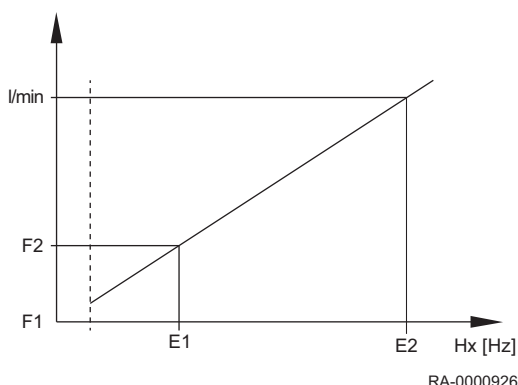
Obr.39 Příklad dvou různých křivek čidel
