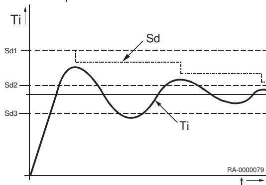
Obr.35 Spínací rozdíl
