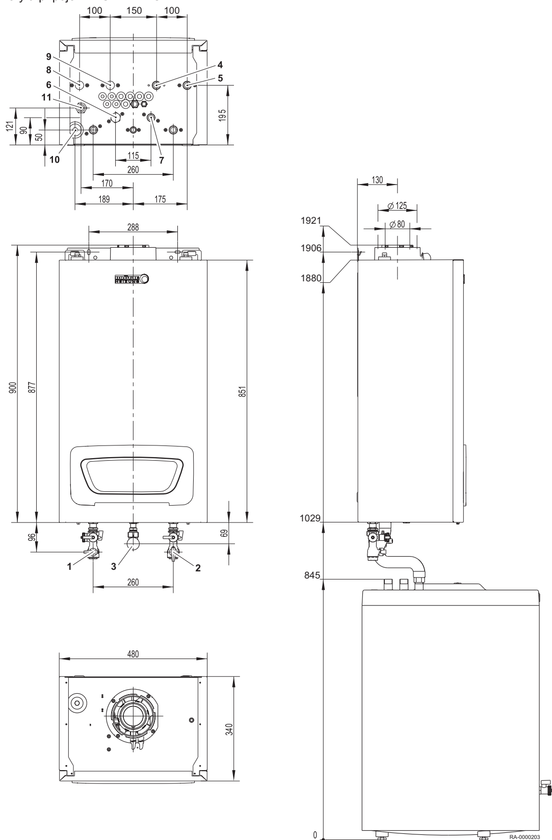
Obr.4 Rozměry a připojení WGB-M EVO
