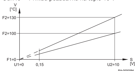
Obr.40 Příklad požadavku na teplo 10 V
