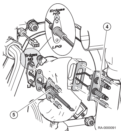
Obr.43 Demontáž zapalovací elektrody a ionizační sondy
