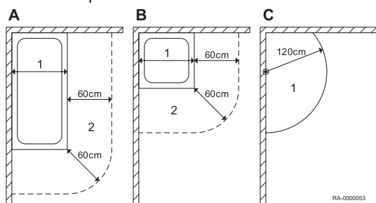
Obr.10 Volné prostory v koupelně a ve sprše
