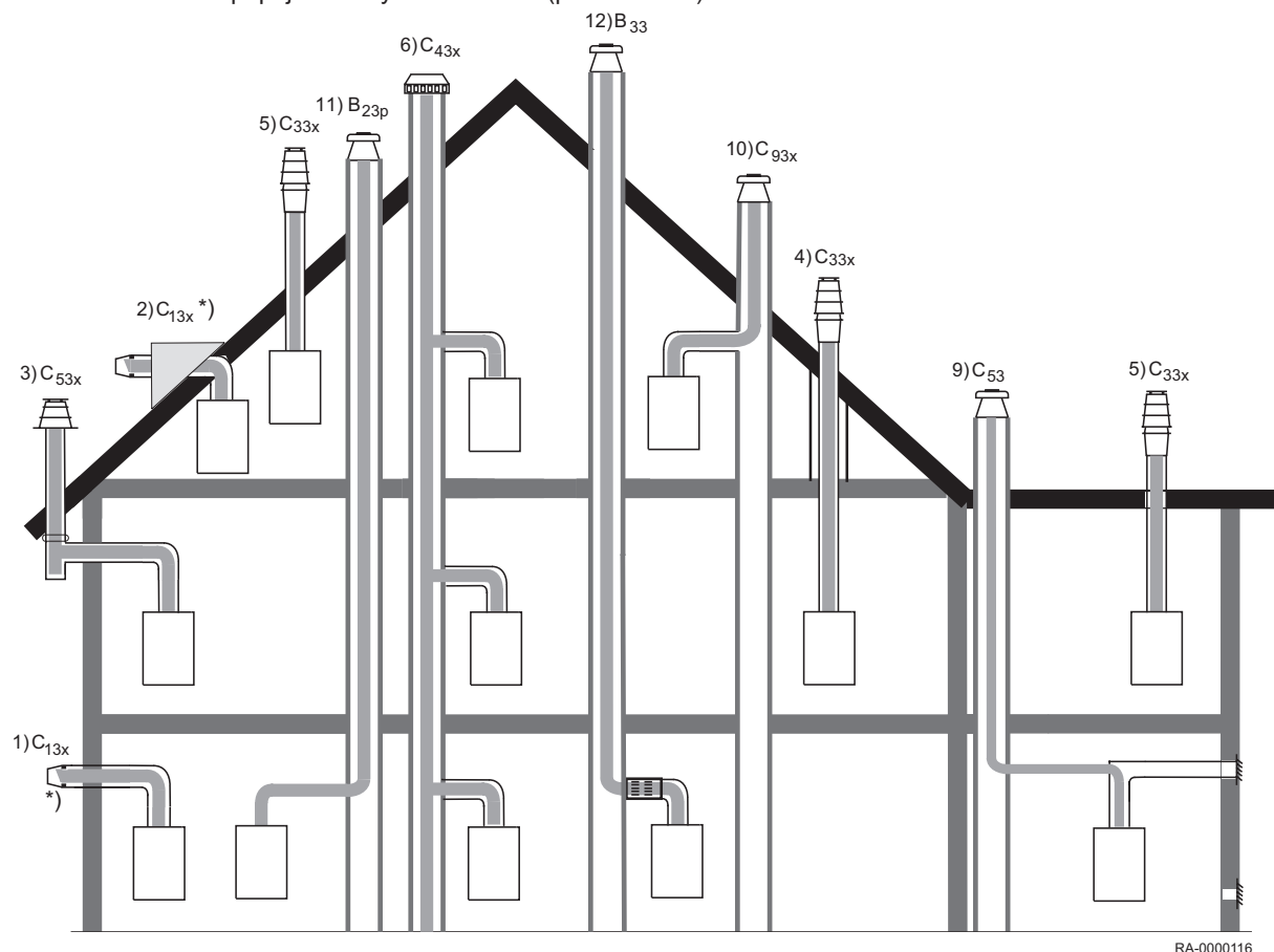
Obr.13 Možnosti připojení se systémem KAS (příslušenství)
