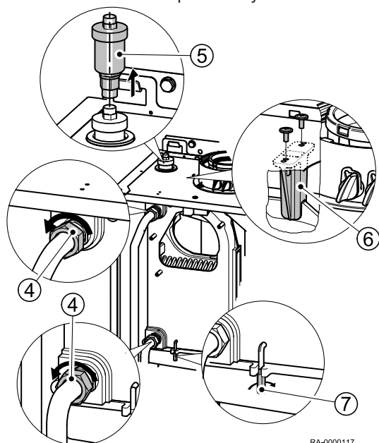
Obr.45 Demontáž tepelného výměníku
