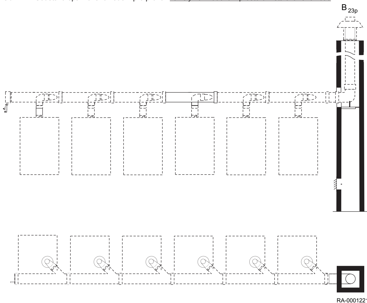
Obr.17 Soustava spalinového vedení pro provoz závislý na vzduchu z prostoru instalovaného kotle
