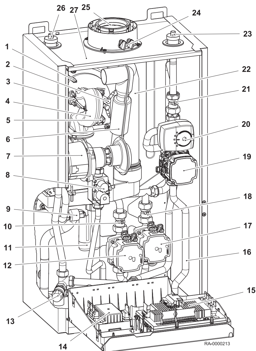
Obr.6 Náhled na kotel WGB-M EVO (zobrazení bez přední stěny a krytu regulační jednotky)
