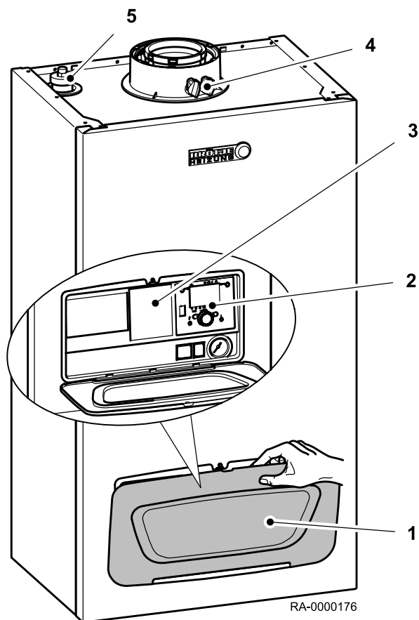
Obr. 1: Výkres celkového uspořádání WBS / WBC
