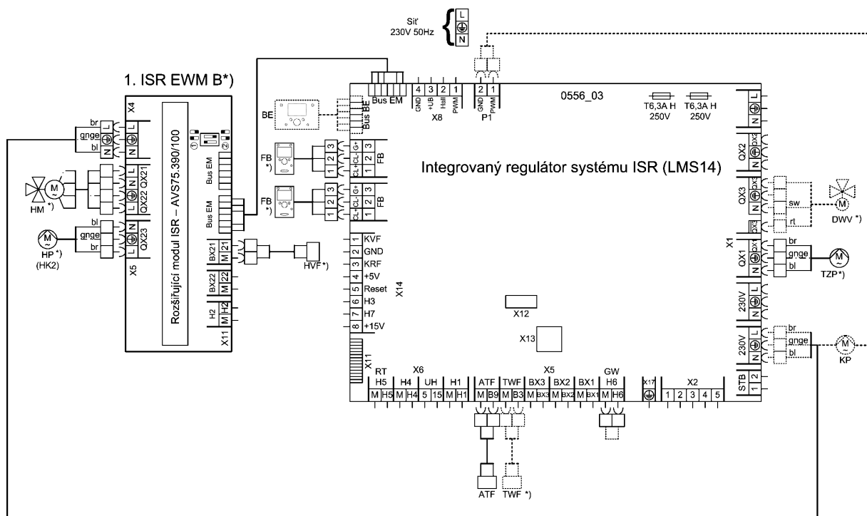
Obr. 7: Schéma připojení
