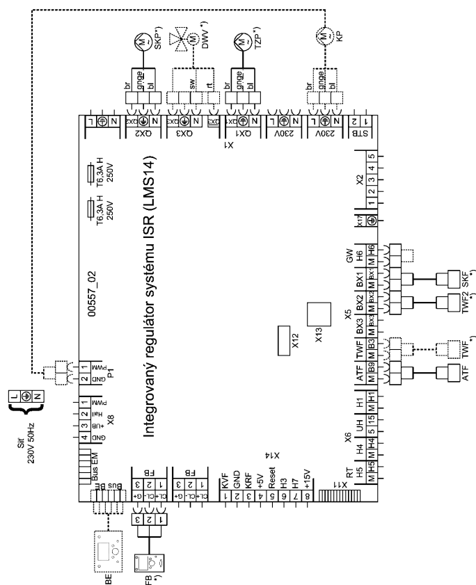
Obr. 9: Schéma připojení
