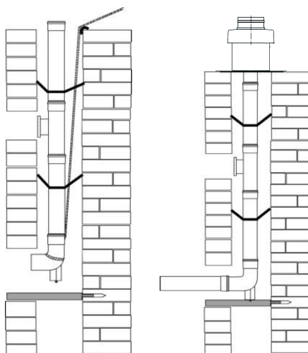
Obr. 12: Zavedení do šachty
