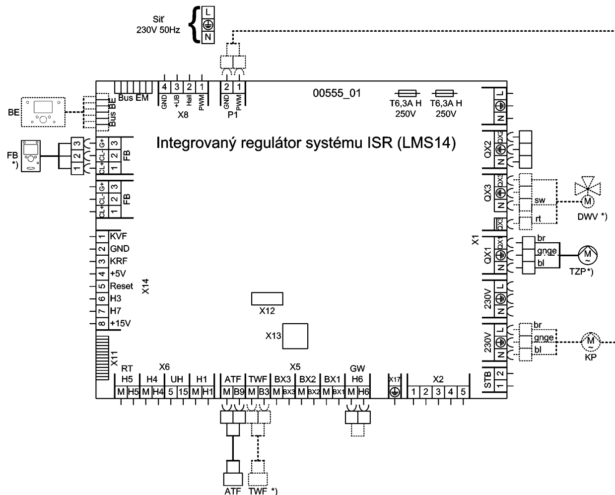
Obr. 5: Schéma připojení
