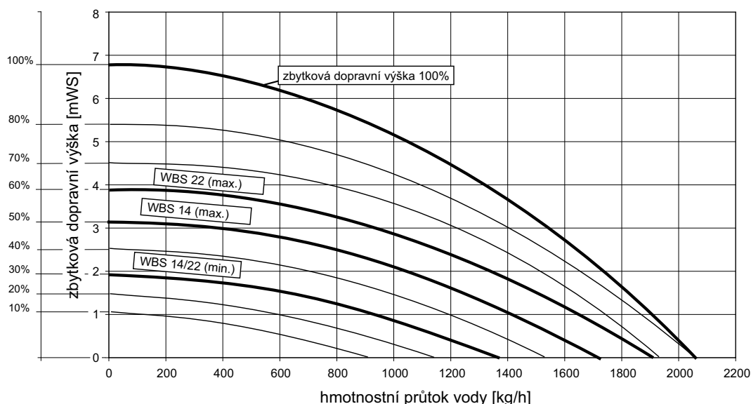
Obr. 24: Zbytková dopravní výška WBS 14/22 H
