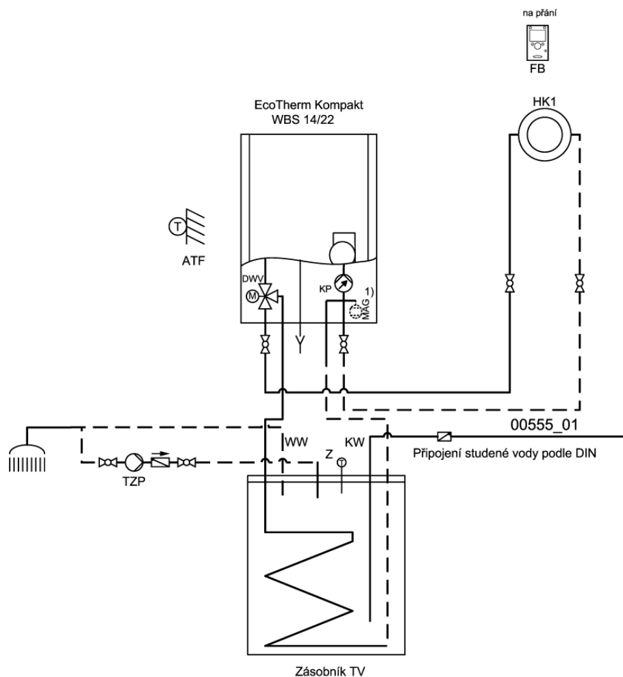
Obr. 4: Příklad použití: Topný okruh s čerpadlem a prostorovým termostatem, včetně regulace teploty zásobníku
