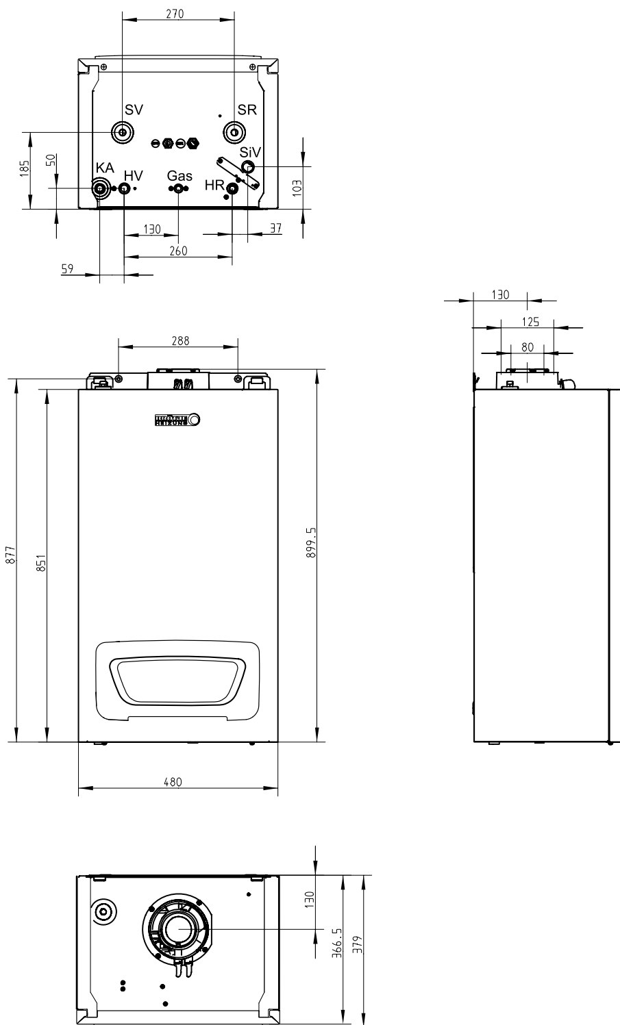
Obr. 1: Rozměry a přípojky kotle
