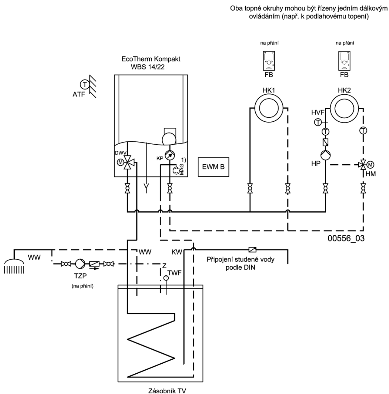
Obr. 6: Příklad použití: 2 topné okruhy s čerpadlem a prostorovým termostatem, včetně regulace teploty zásobníku
