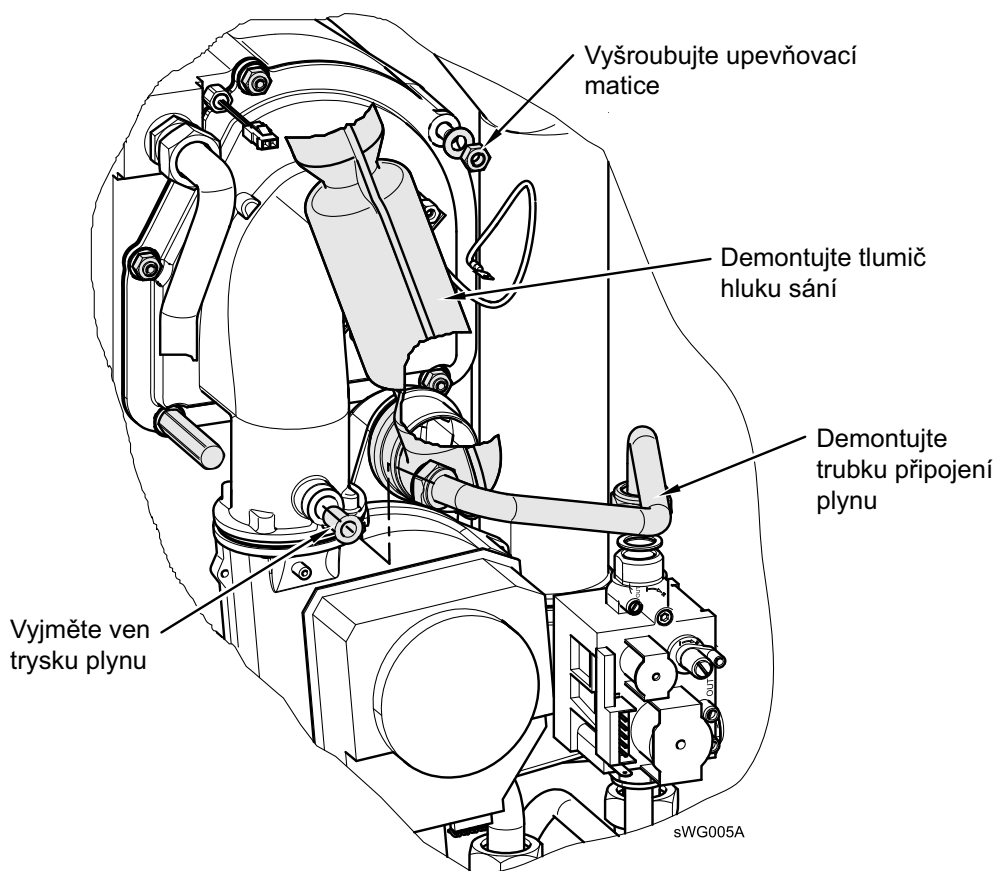
Obr. 30: Demontáž plynového hořáku
