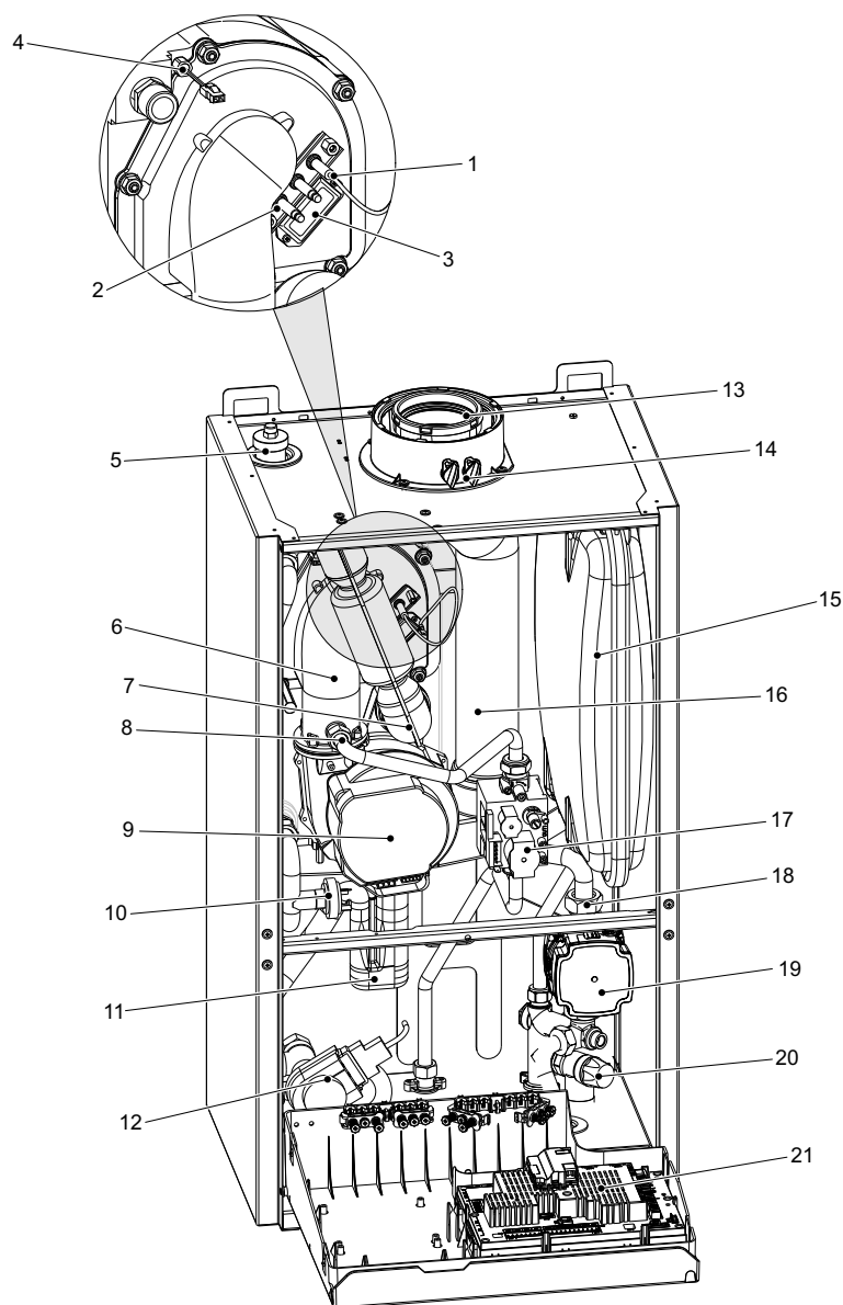
Obr. 31: Zobrazení kotle WBS (bez přední stěny a krytu regulace)
