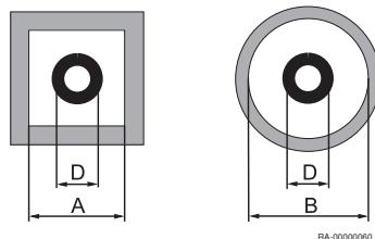
Obr.19 Minimální rozměry kouřovodu
