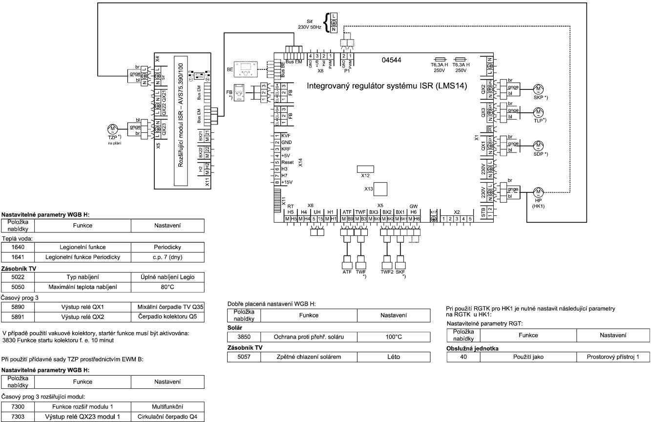
Obr.14 Schéma zapojení
