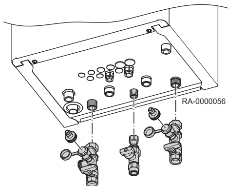
Obr. 17 Instalace uzavíracích kohoutů
