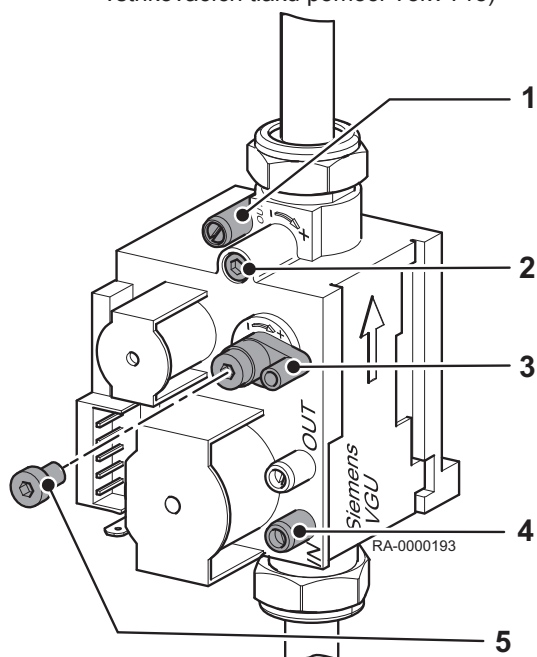
Obr.21 Plynový ventil (nastavení vstřikovacích tlaků pomocí Torx T15)
