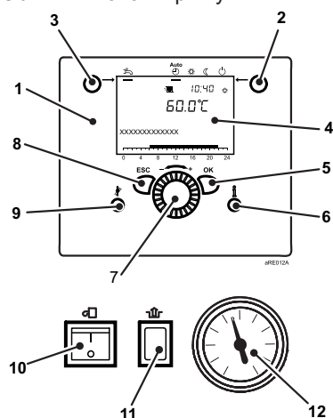
Obr.7 Provozní prvky
