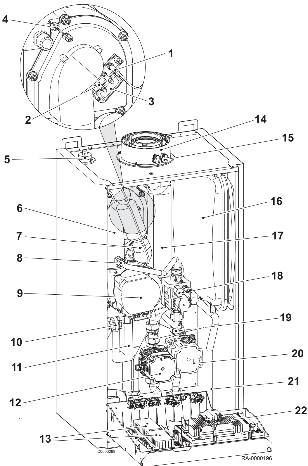
Obr.5 Náhled na kotel WGB (zobrazení bez přední stěny a krytu regulační jednotky)
