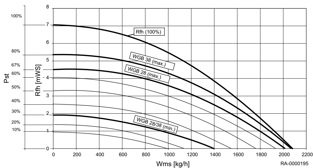
Obr.2 Celkový dynamický spád WGB 28 — 38
