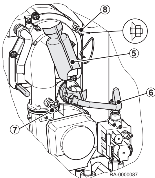
Obr.40 Demontáž hořáku
