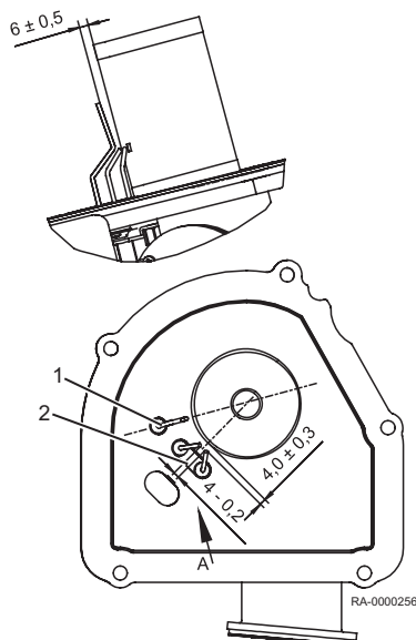
Obr.39 Elektrody
