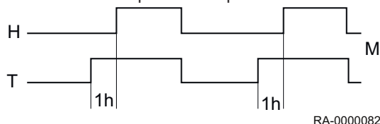
Obr.35 Doba napouštění dopředu
