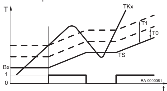
Obr.34 Naplňování zásobníku
