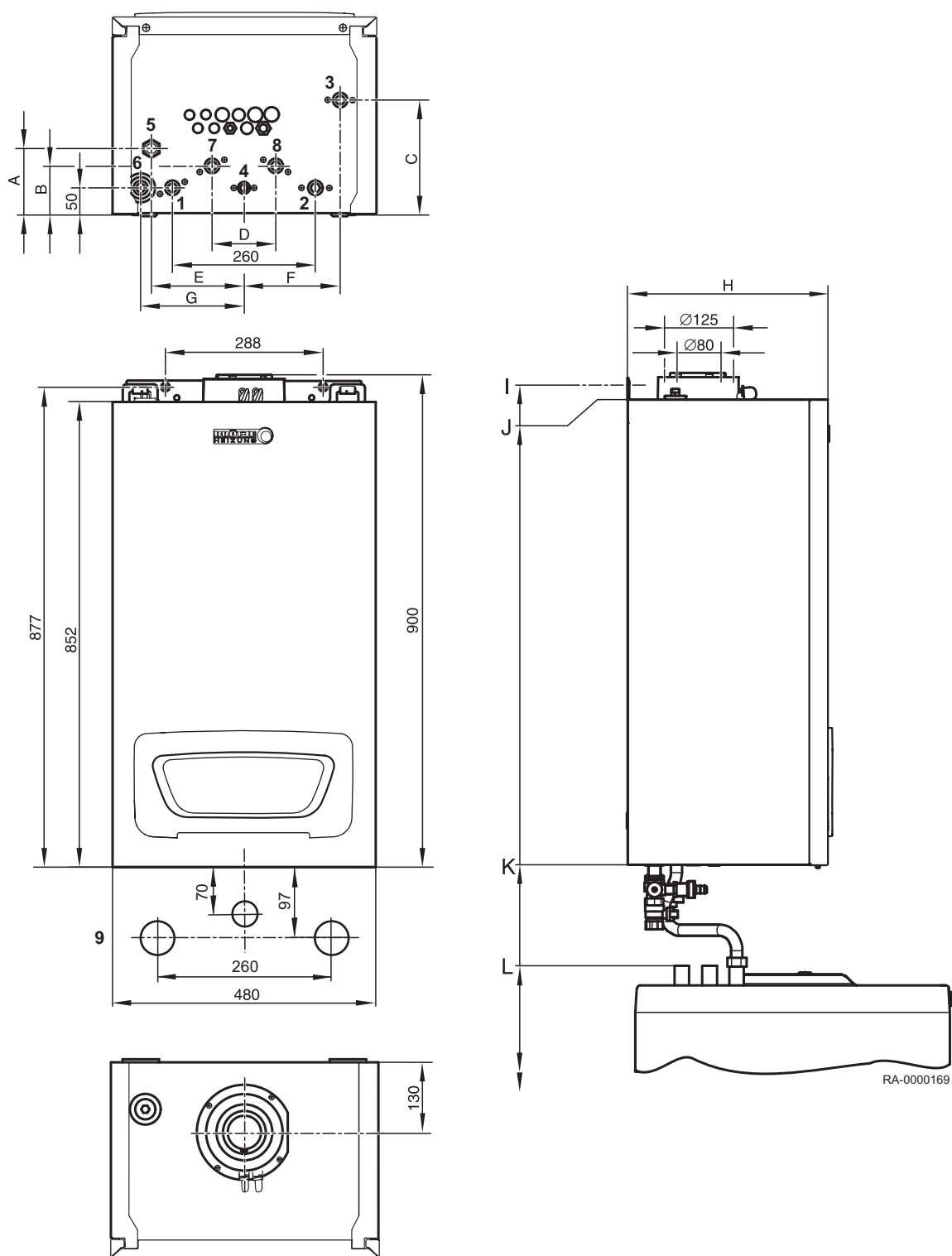
Obr.3 Rozměry a zapojení WGB
