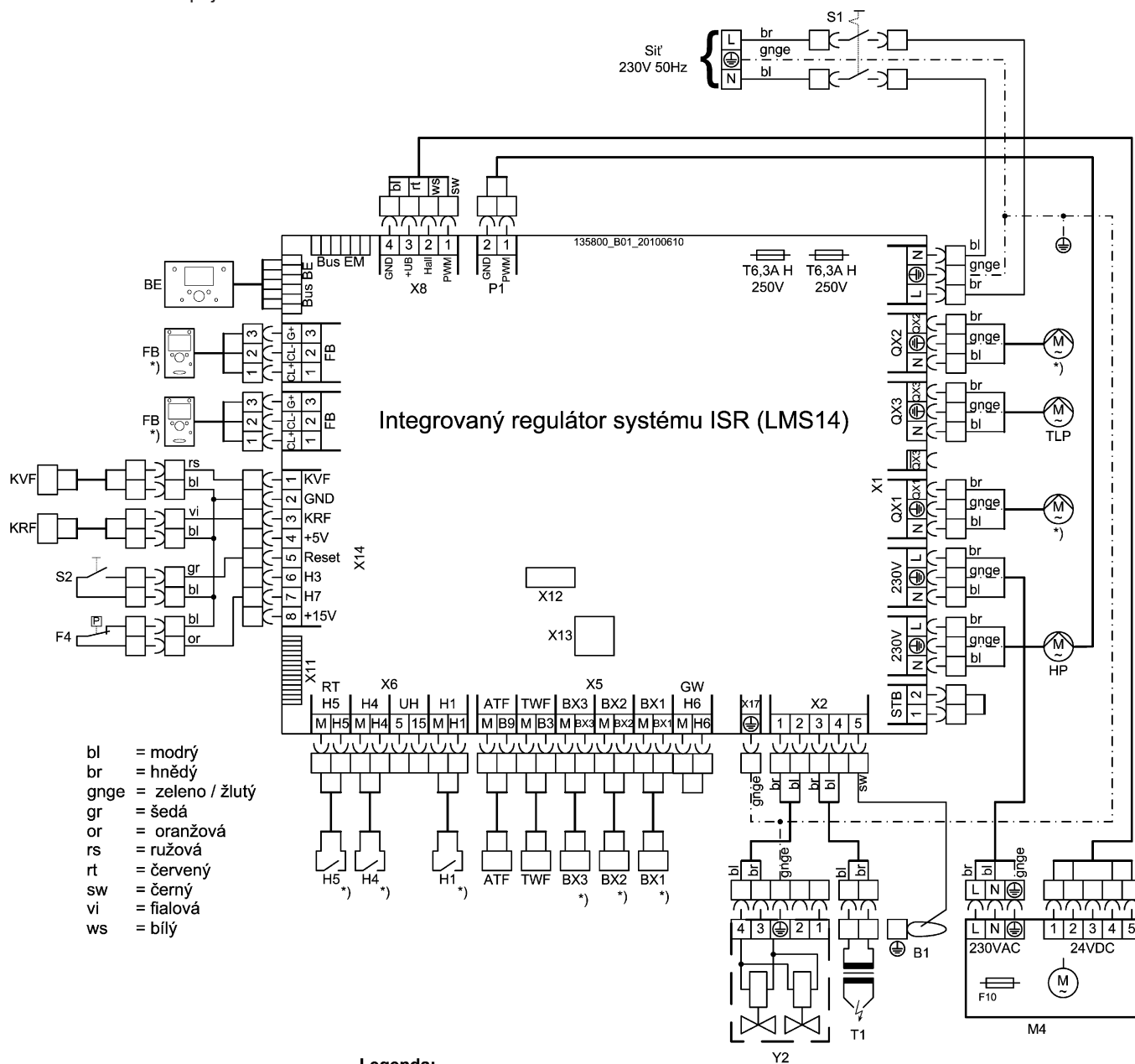
Obr.4 Schéma zapojení
