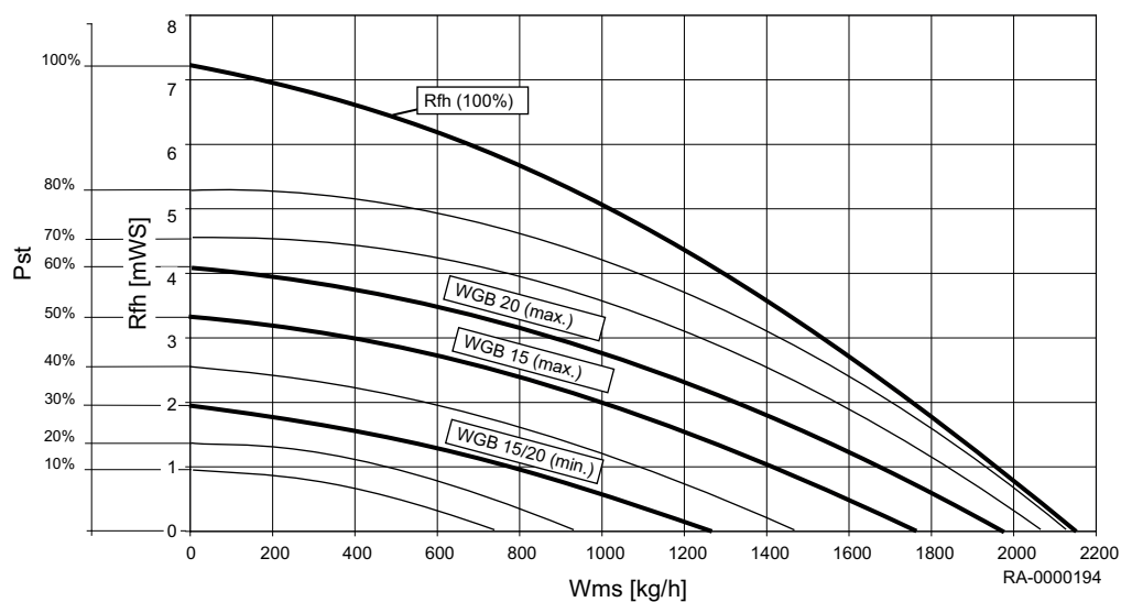
Obr.1 Celkový dynamický spád WGB 15 — 20
