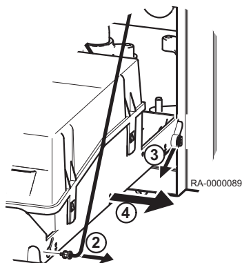
Obr.38 Sejmutí ovládacího panelu
