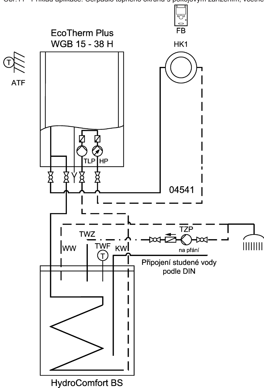
Obr.11 Příklad aplikace: Čerpadlo topného okruhu s pokojovým zařízením, včetně regulace teploty zásobníku
