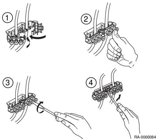
Obr.20 Uvolnění napětí
