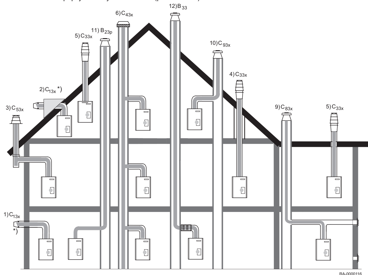
Obr.18 Možnosti připojení se systémem KAS (příslušenství)
