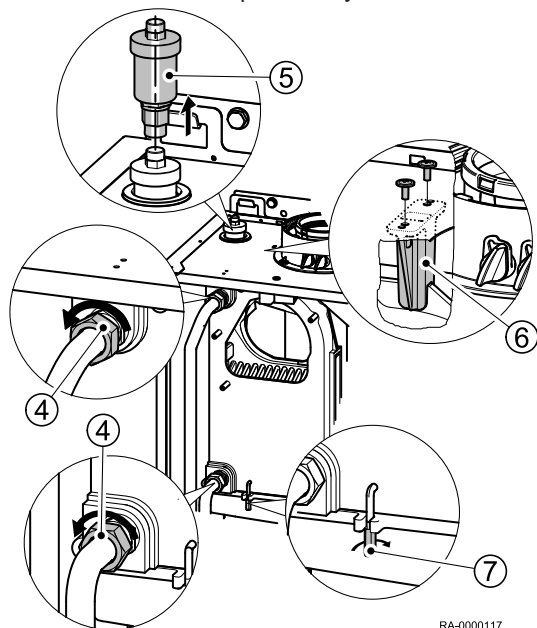
Obr.41 Demontáž tepelného výměníku.
