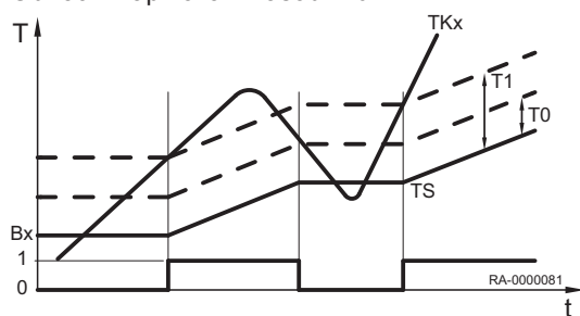
Obr.30 Naplňování zásobníku
