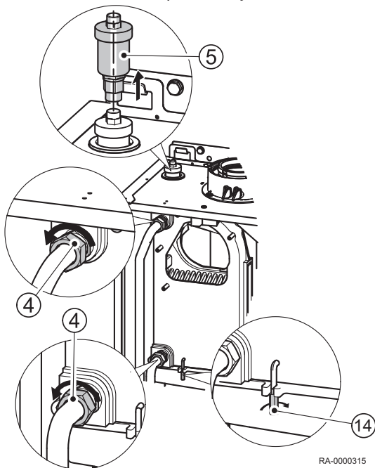
Obr.37 Demontáž tepelného výměníku.
