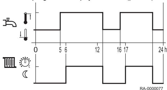
Obr.27 Uvolnění dle programu časového sepnutí 4 (příklad)
