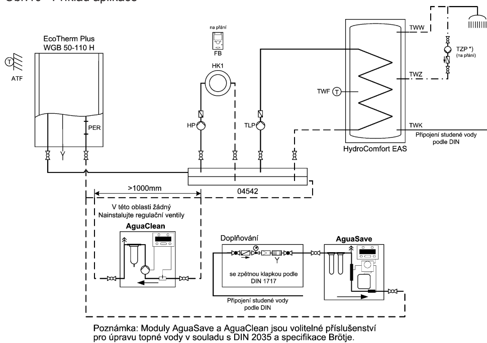
Obr.10 Příklad aplikace
