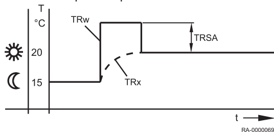
Obr.22 Podpůrné topení
