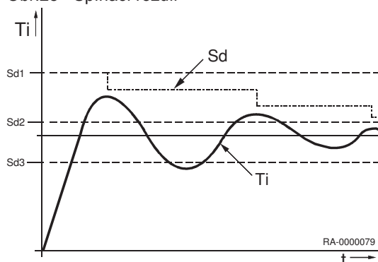
Obr.28 Spínací rozdíl
