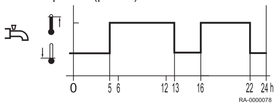
Obr.27 Uvolnění dle programu časového sepnutí 4 (příklad)
