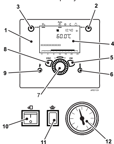
Obr.6 Provozní prvky
