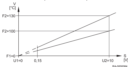
Obr.33 Příklad požadavku na teplo
