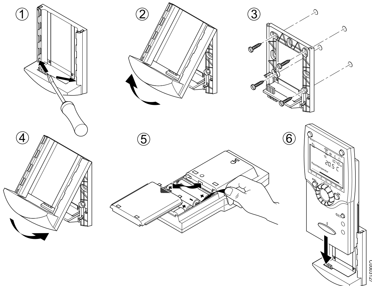
Rys. 7: Montaż regulatora pokojowego RGTF/RGTKF
