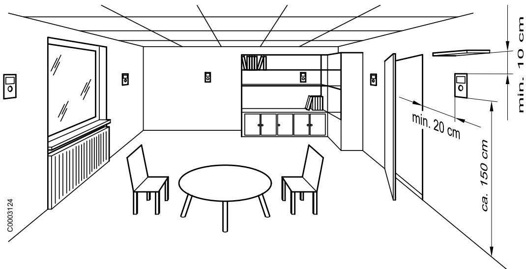
Abb. 5: Montageort (Montagebeispiele)
