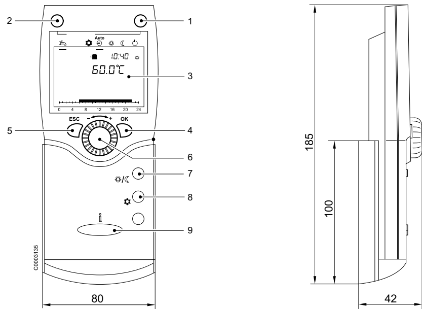
Abb. 1: Übersicht und Abmessungen
