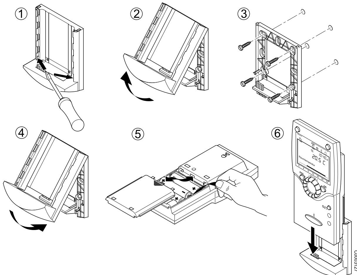
Abb. 7: Montage des Raumgerätes RGTF/RGTKF
