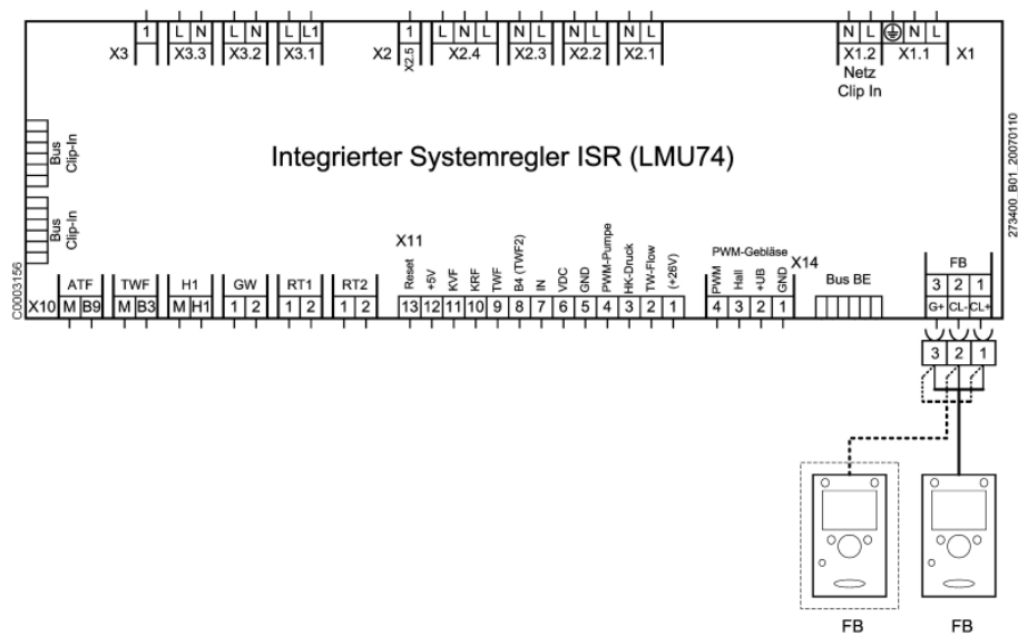
Fig. 3: Schema elettrico per il collegamento al regolatore di sistema ISR-LMU (a partire da LMU 74)
