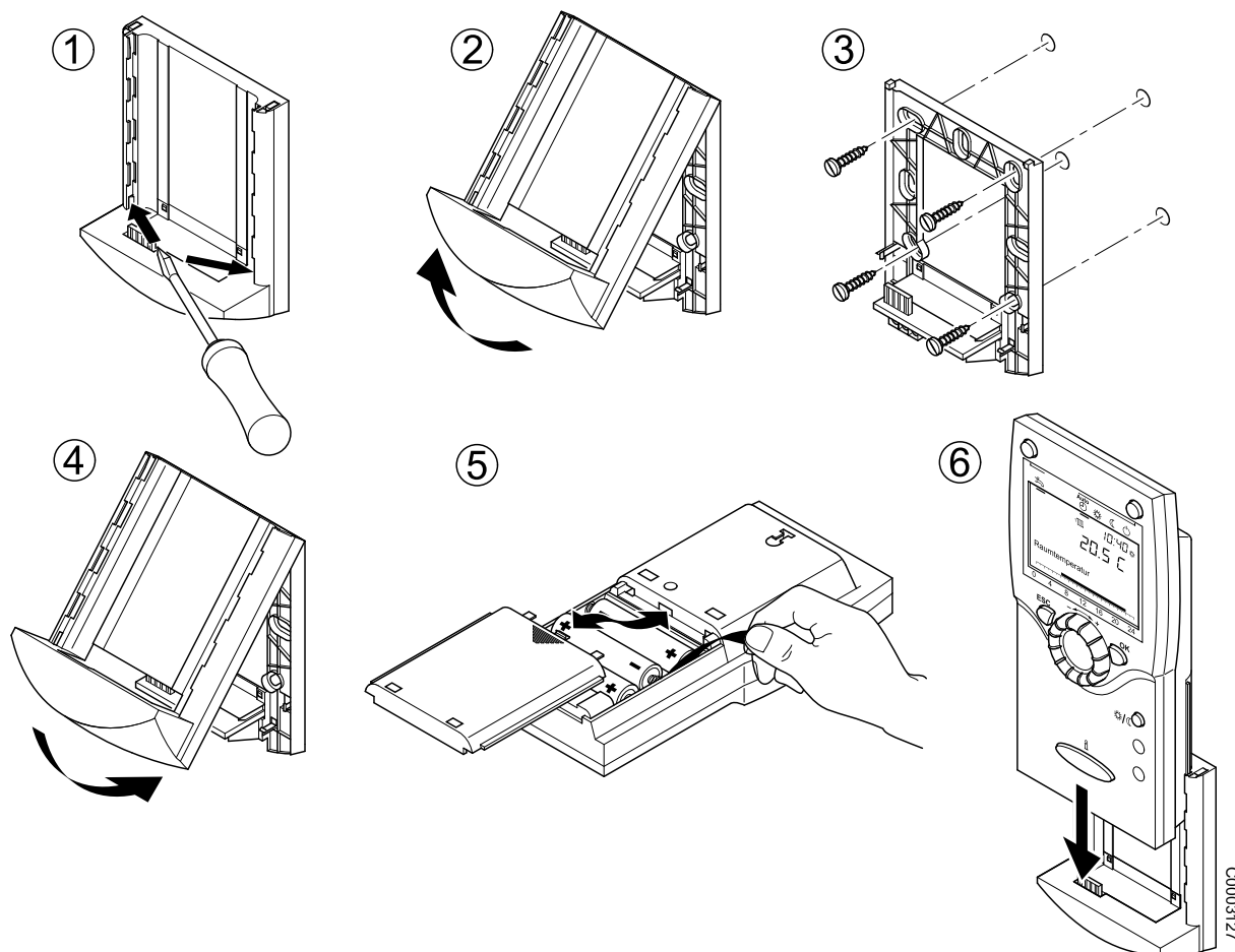
Obr. 7: Montáž termostatu RGTF/RGTKF
