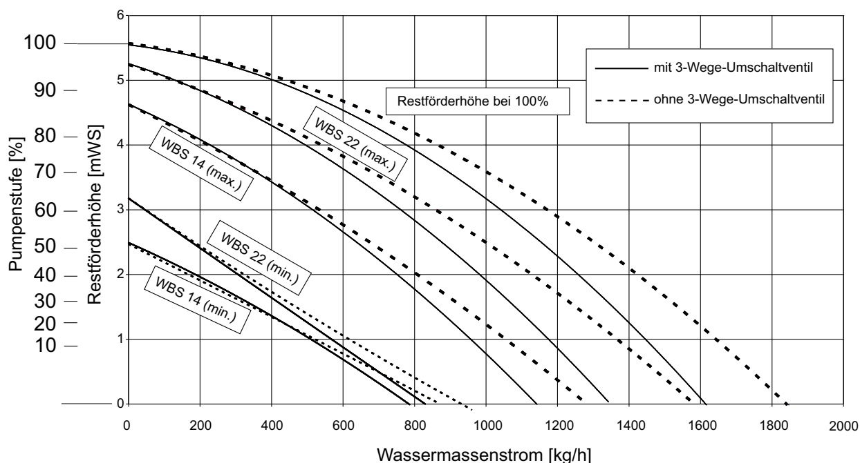
Obr. 25: Zbytková čerpací výška WBS 14/22 E
