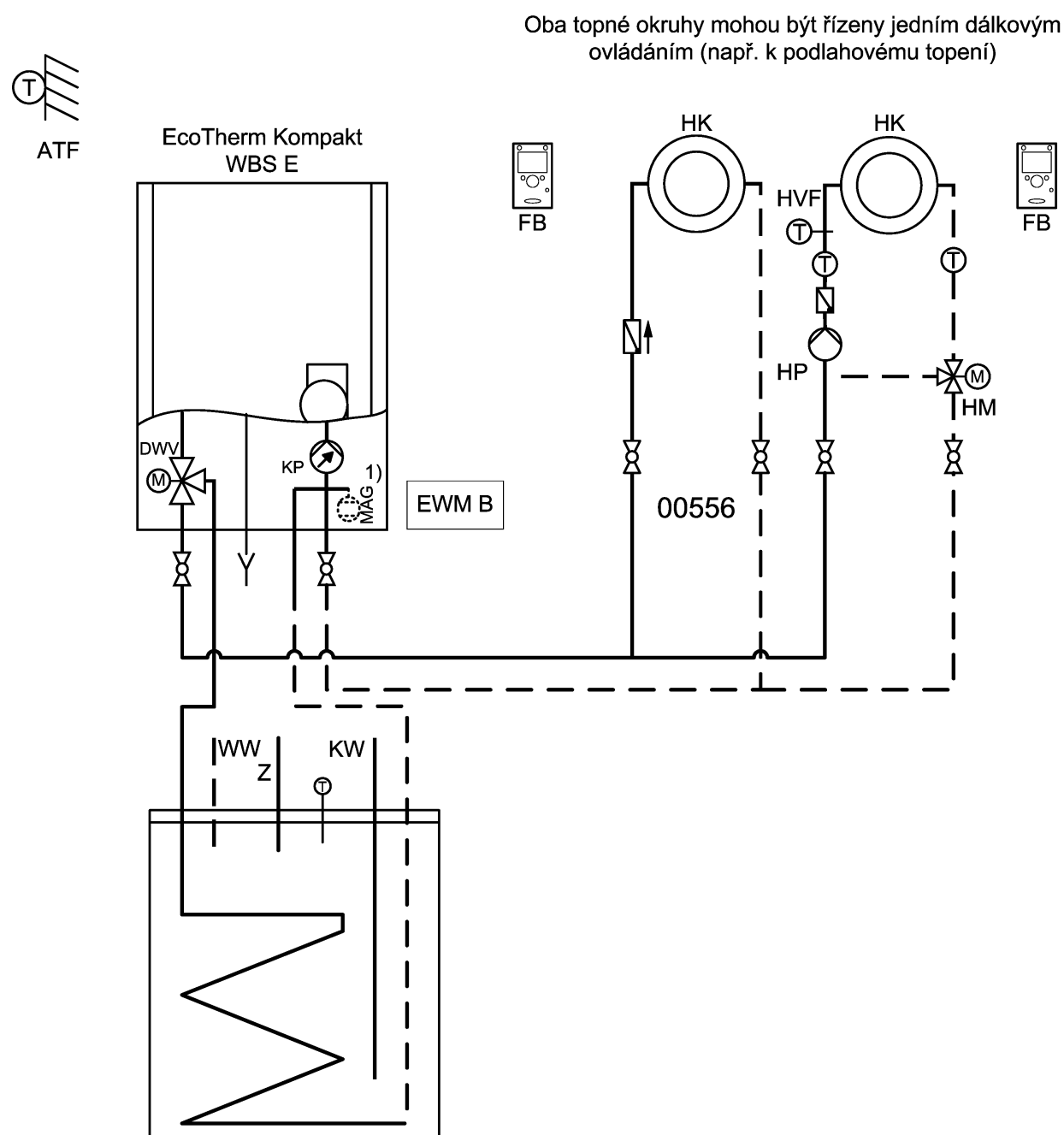
Obr. 6: Příklad použití: 2 topné okruhy s čerpadlem a prostorovým termostatem, včetně regulace teploty zásobníku
