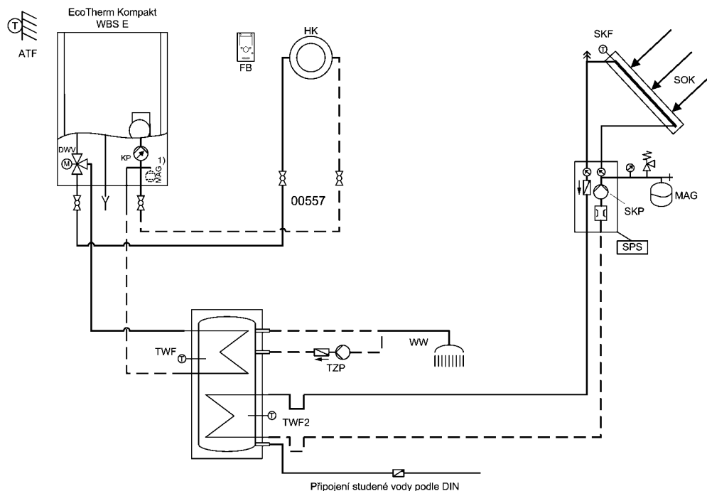
Obr. 8: Příklad použití: Topný okruh s čerpadlem a prostorovým termostatem a solárním zásobníkem
