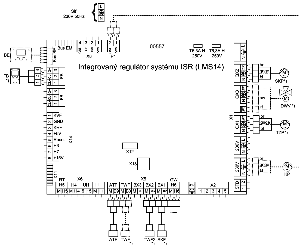
Obr. 9: Schéma připojení
