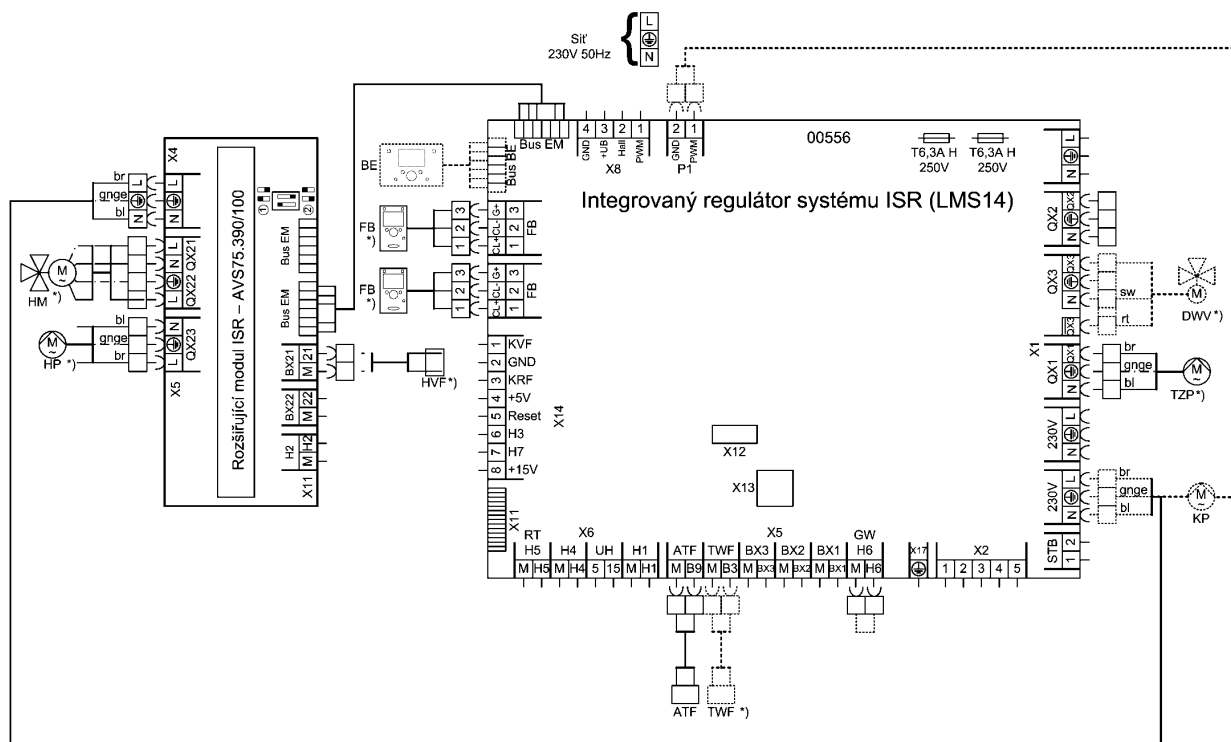
Obr. 7: Schéma připojení
