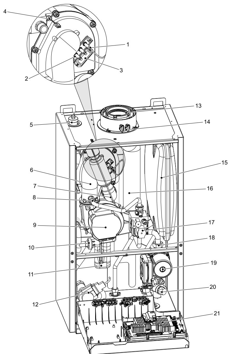
Obr. 32: Zobrazení kotle WBS (bez přední stěny a krytu regulace)
