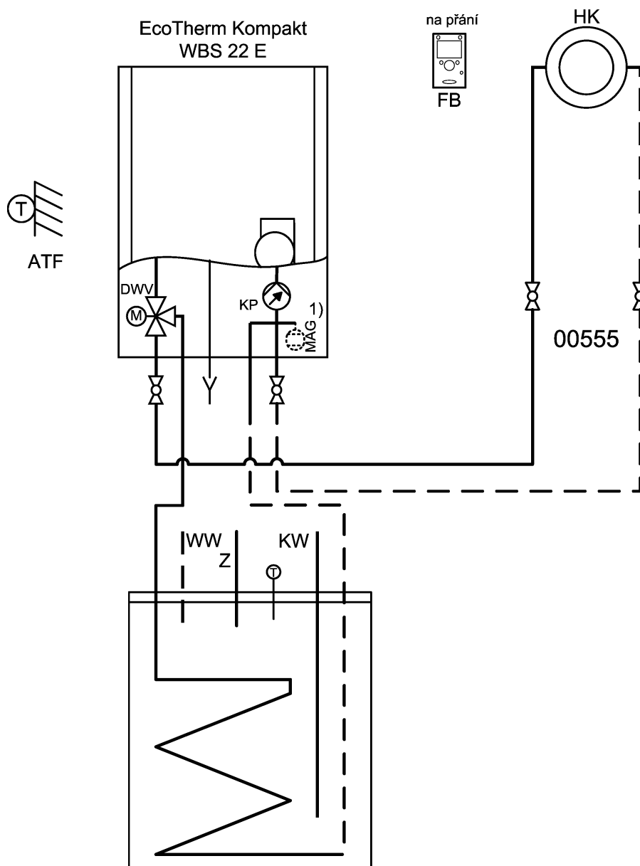
Obr. 4: Příklad použití: Topný okruh s čerpadlem a prostorovým termostatem, včetně regulace teploty zásobníku
