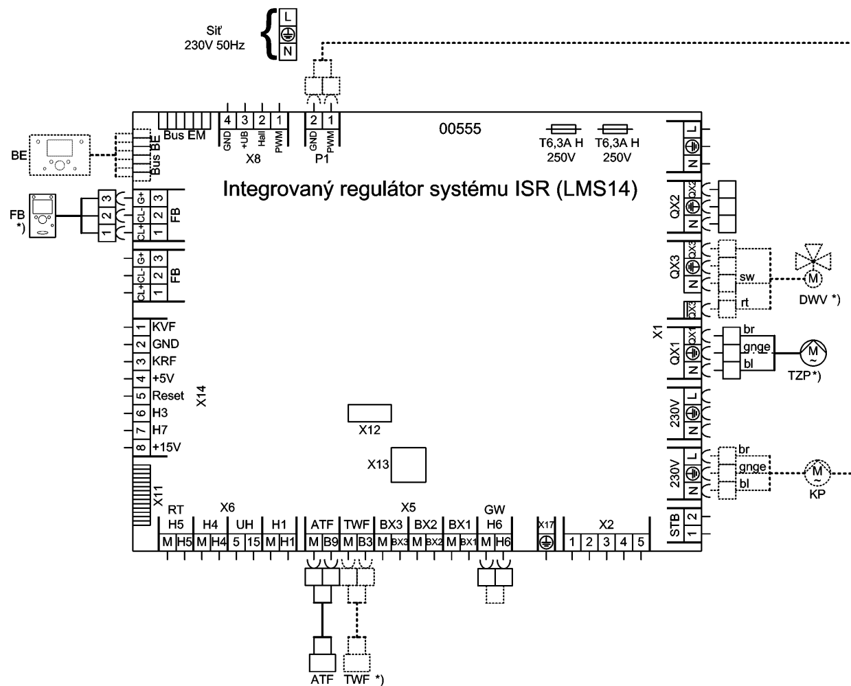
Obr. 5: Schéma připojení
