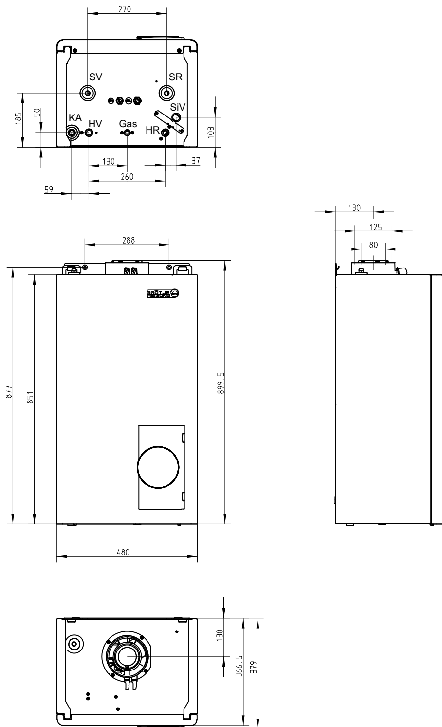
Obr. 1: Rozměry a přípojky kotle
