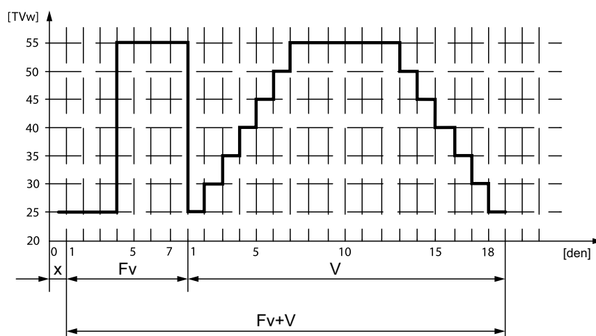
Obr. 25: Teplotní profil při funkci vysoušení podlahy
