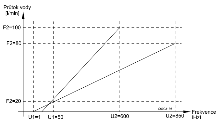
Obr. 31: Příklad pro dvě různé křivky
