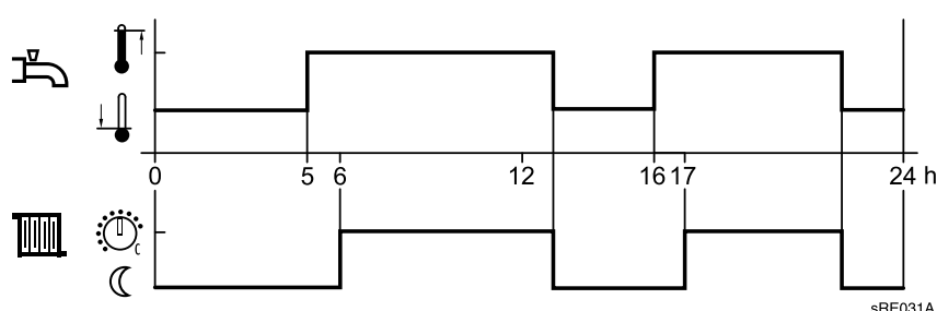
Obr. 27: Uvolnění v závislosti na programech časového spínání topných okruhů (příklad)
