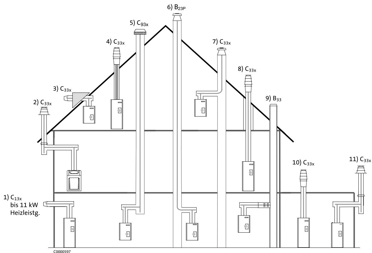
Obr. 11: Možnosti připojení se systémem KAS 80 (příslušenství)
