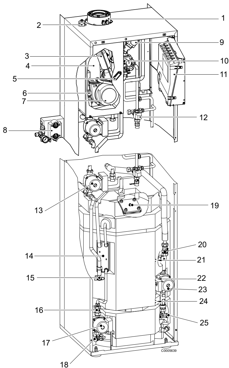
Obr. 35: Pohled na kotel (zobrazeno bez přední stěny)
