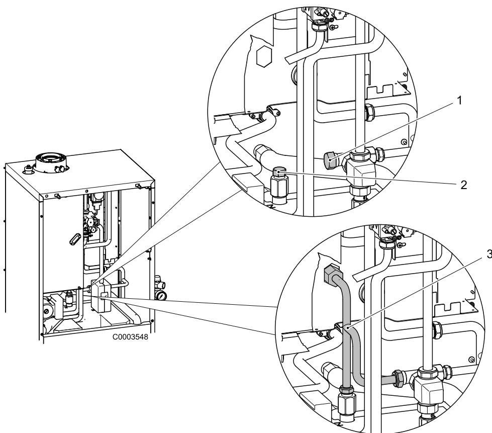
Obr. 9: Montáž cirkulační trubky (nepovinná)
