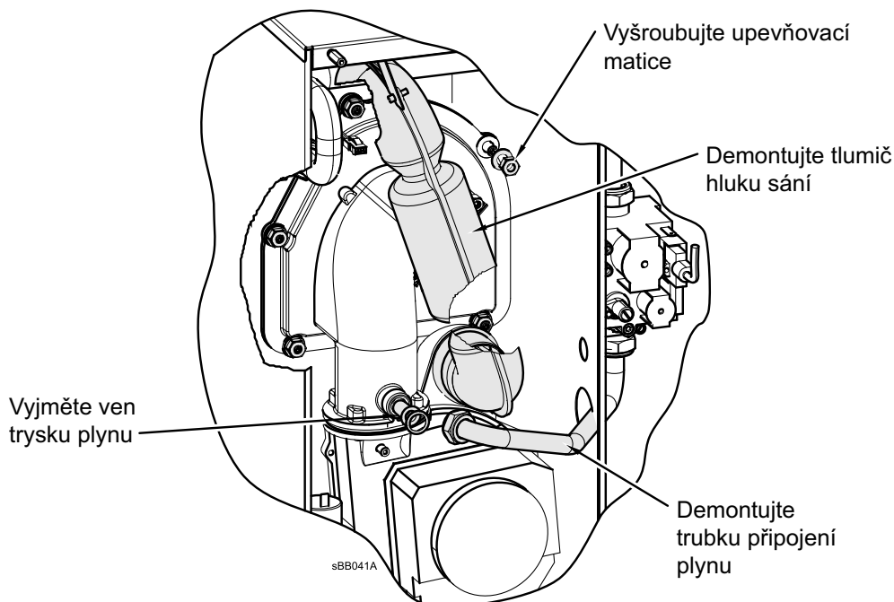
Obr. 34: Demontáž plynového hořáku
