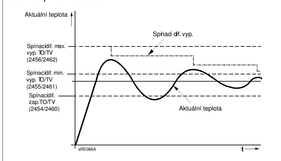
Obr. 29: Spínací difference
