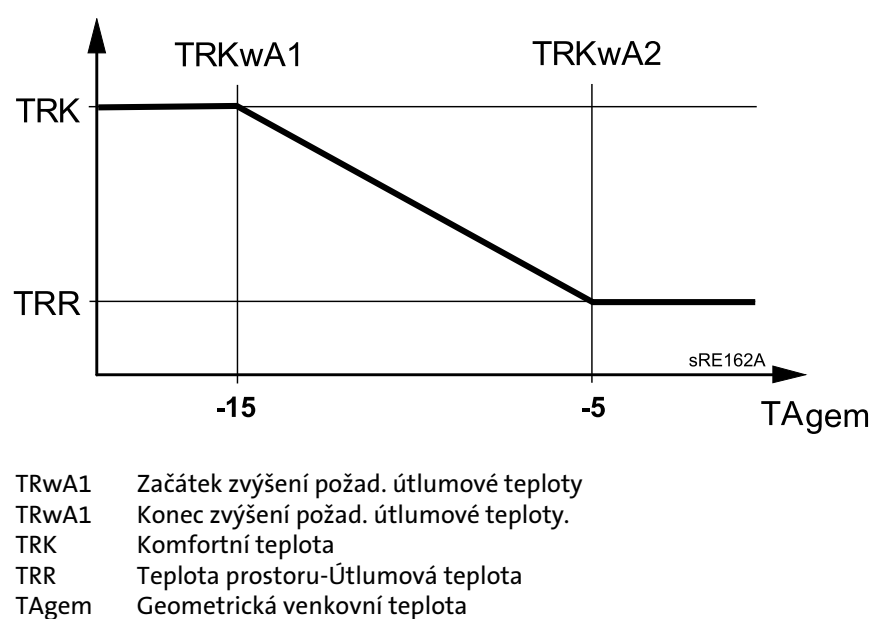
Obr. 24: Zvýšení požad. útlumové teploty
