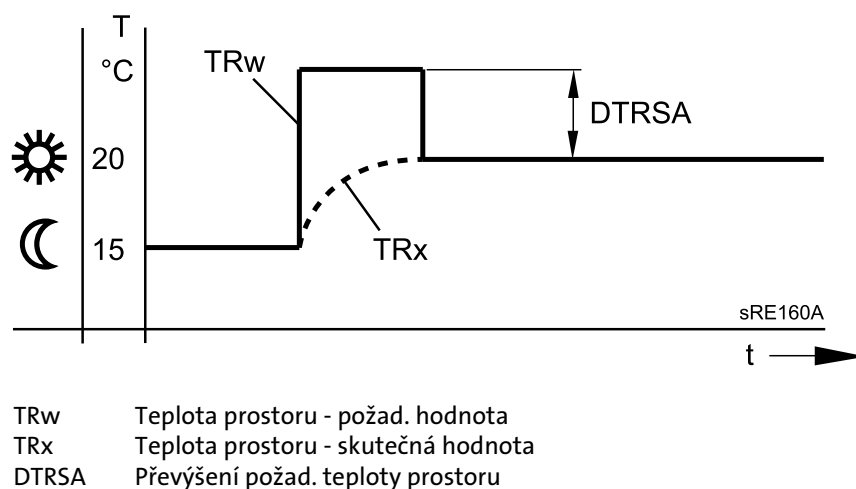
Obr. 22: Rychlé natopení
