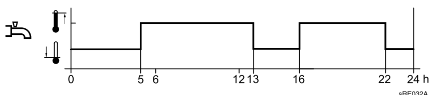
Obr. 28: Uvolnění podle časového programu 4 (příklad)
