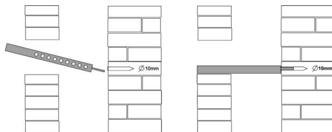
Obr. 12: Montáž opěrné lišty
