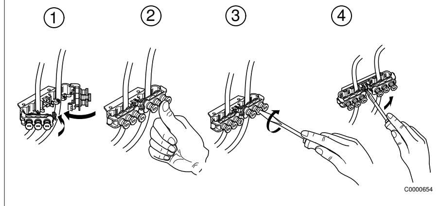
Obr. 16: Prvek odlehčení tahového pnutí
