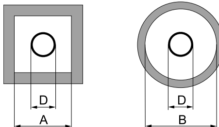
Obr. 14: Minimální rozměry šachty
