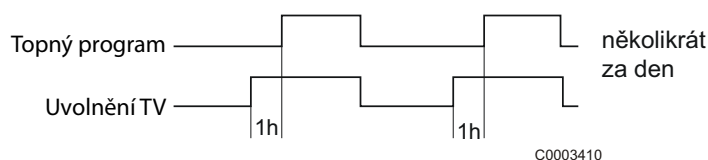
Obr. 30: Předstih nabíjení
