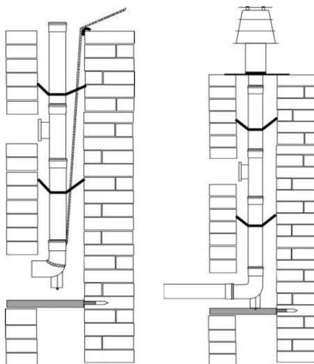
Obr. 13: Zavedení do šachty
