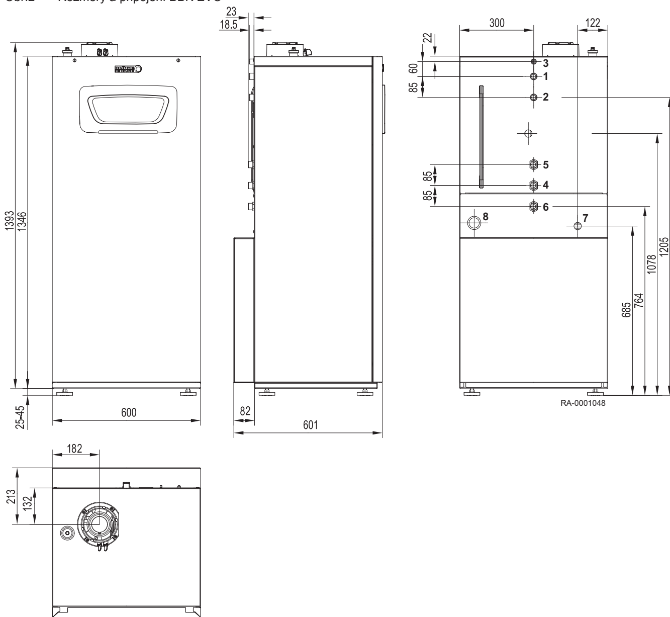
Obr.2 Rozměry a připojení BBK EVO
