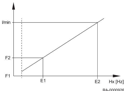
Obr.35 Příklad dvou různých křivek čidel
