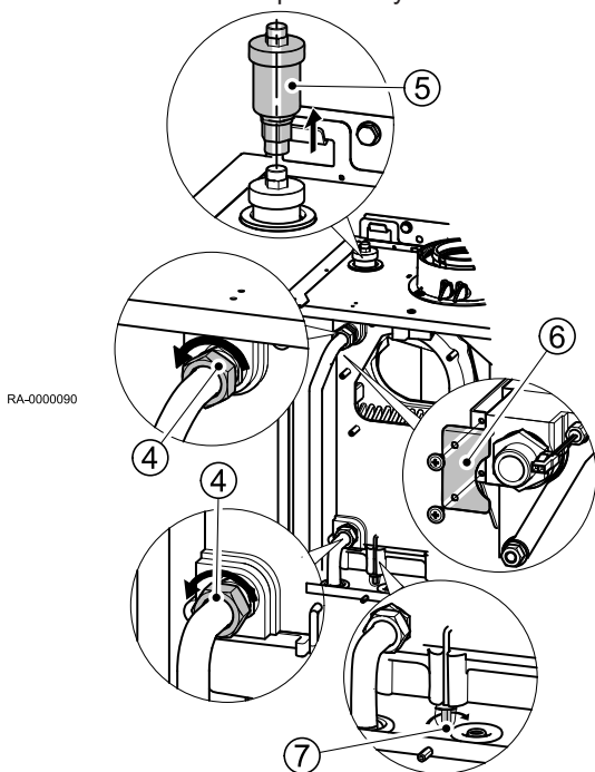
Obr.40 Demontáž tepelného výměníku
