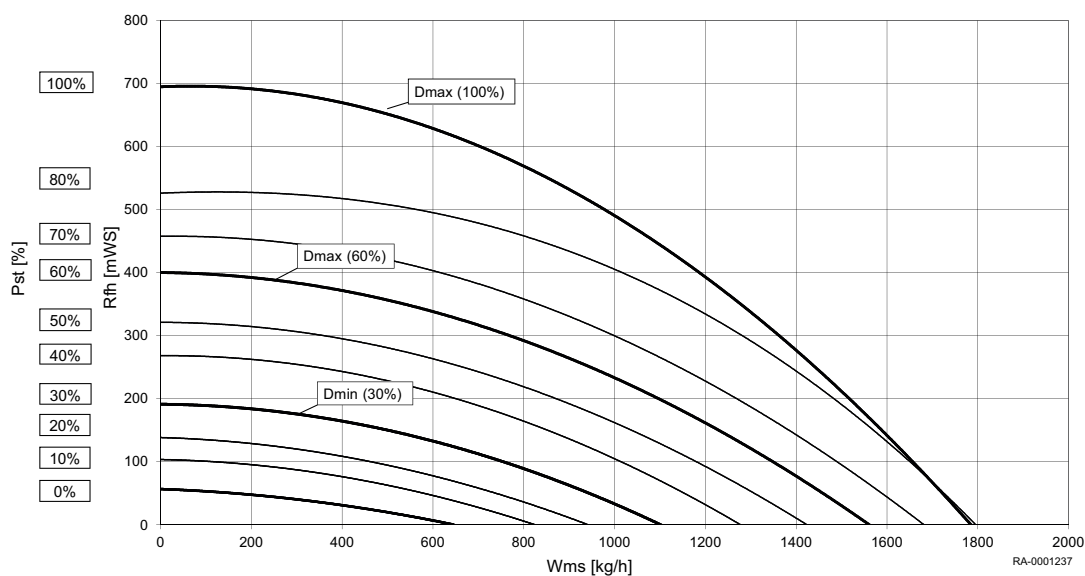
Obr.1 Celkový dynamický spád BBK EVO 20/22
