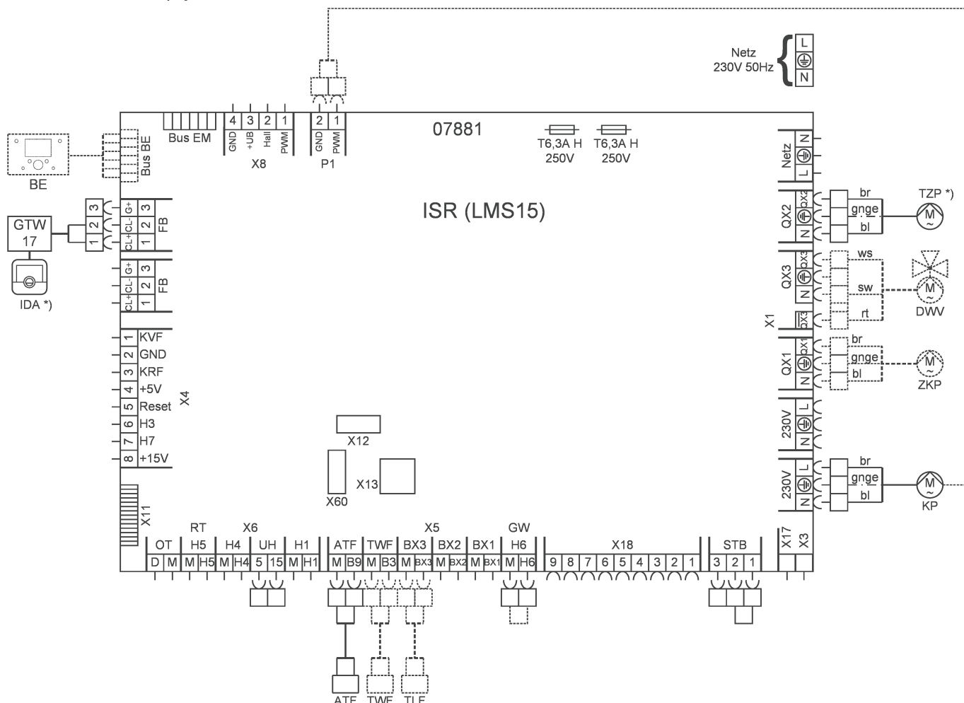
Obr.10 Schéma zapojení
