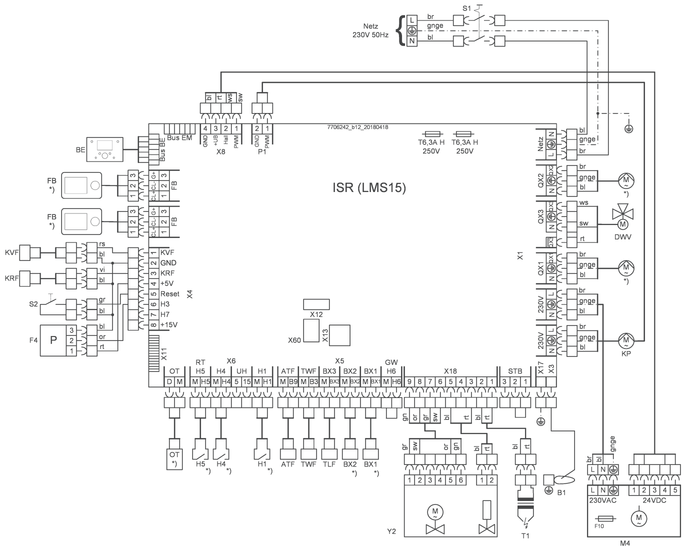
Obr.3 Schéma zapojení BBK EVO
