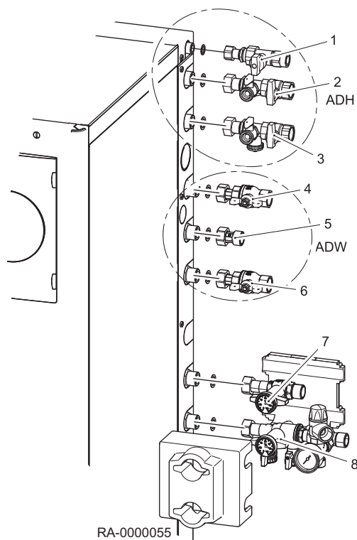
Obr.11 Instalace uzavíracích kohoutů
