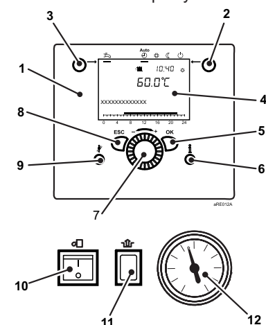
Obr.5 Provozní prvky
