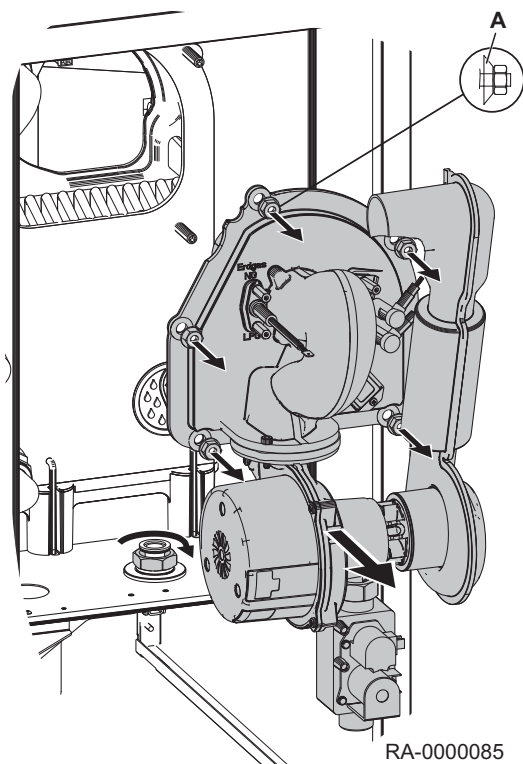
Obr.39 Demontáž hořáku
