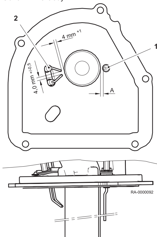
Obr.37 Elektrody
