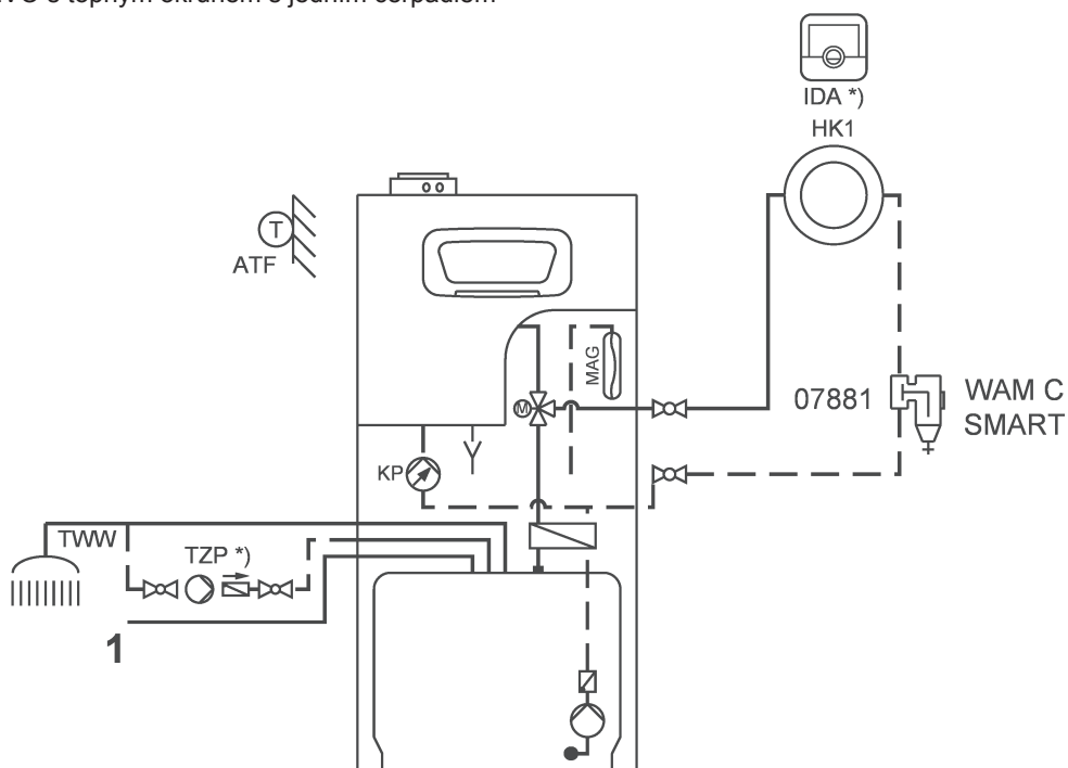
2) Připojení studené vody v souladu s DIN *) volitelně
