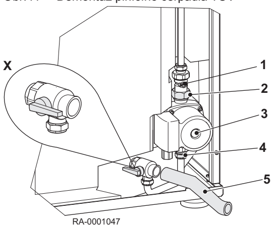
Obr.41 Demontáž plnicího čerpadla TUV
