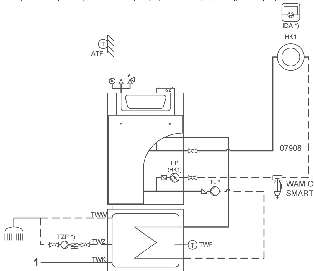
Obr.9 Příklad aplikace: Čerpadlo topného okruhu s pokojovým zařízením, včetně regulace teploty zásobníku
