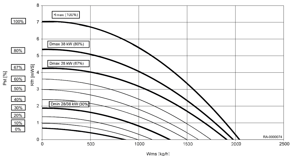
Obr.2 Celkový dynamický spád BGB EVO 28 – 38
