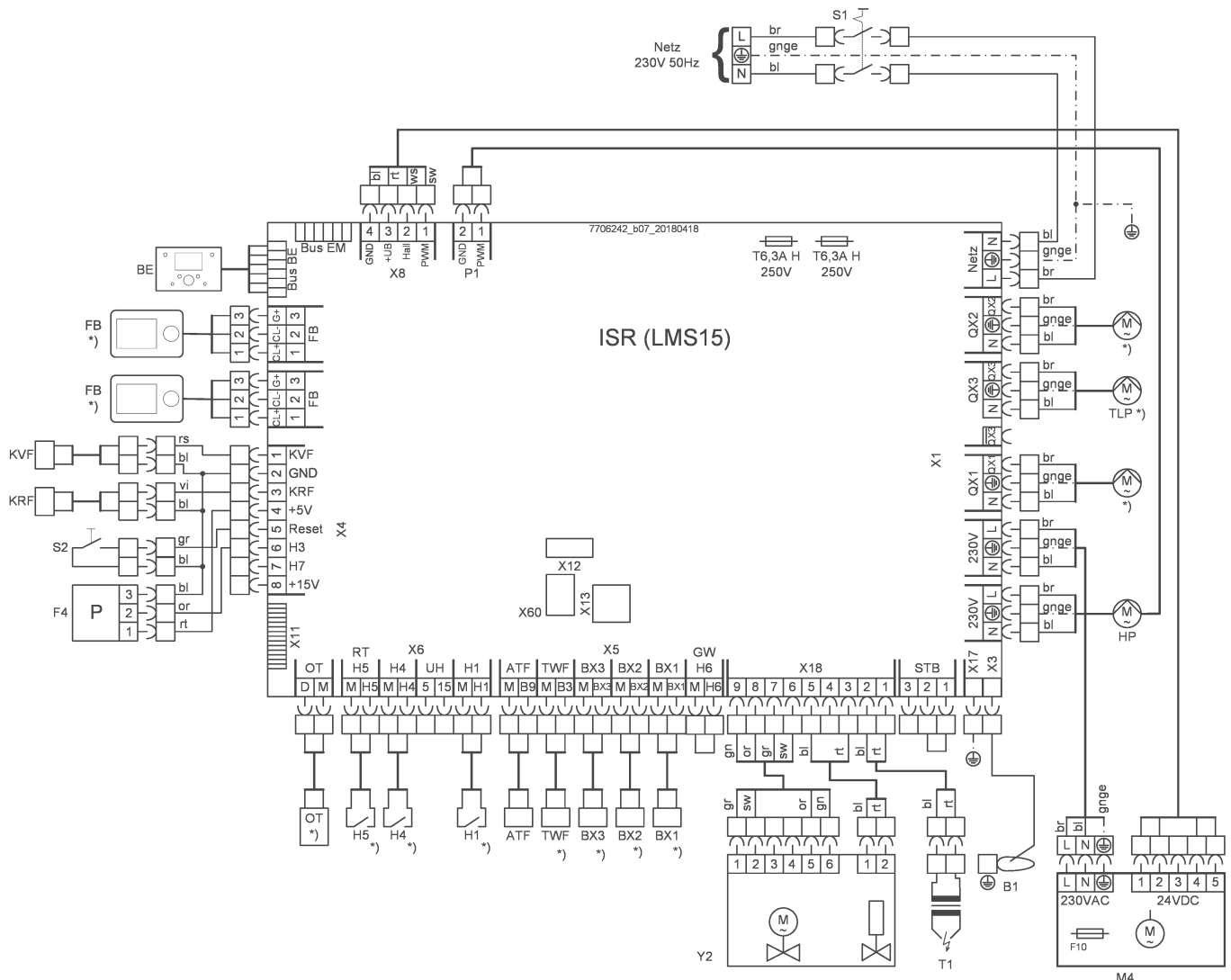
Obr.4 Schéma zapojení BGB EVO 15 – 28
