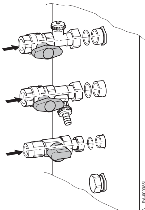
Obr.11 Instalace uzavíracích kohoutů
