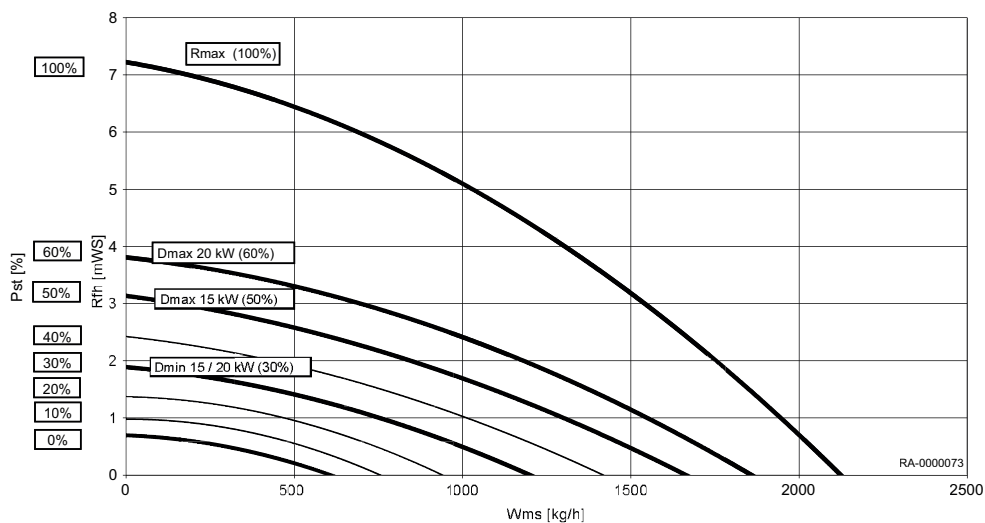
Obr.1 Celkový dynamický spád BGB EVO 15 – 20
