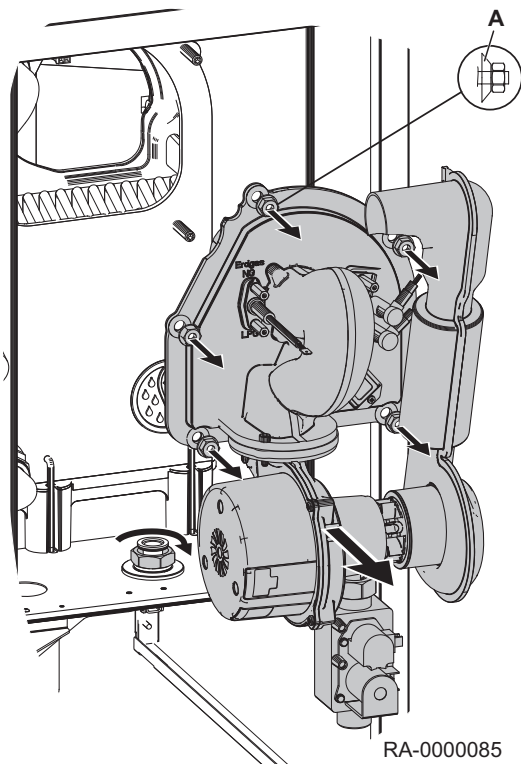
Obr.40 Demontáž hořáku
