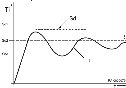
Obr.32 Spínací rozdíl
