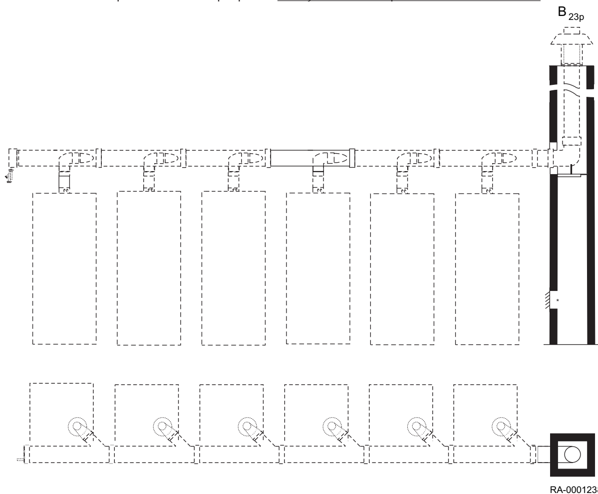
Obr.16 Soustava spalínového vedení pro provoz závislý na vzduchu z prostoru instalovaného kotle
