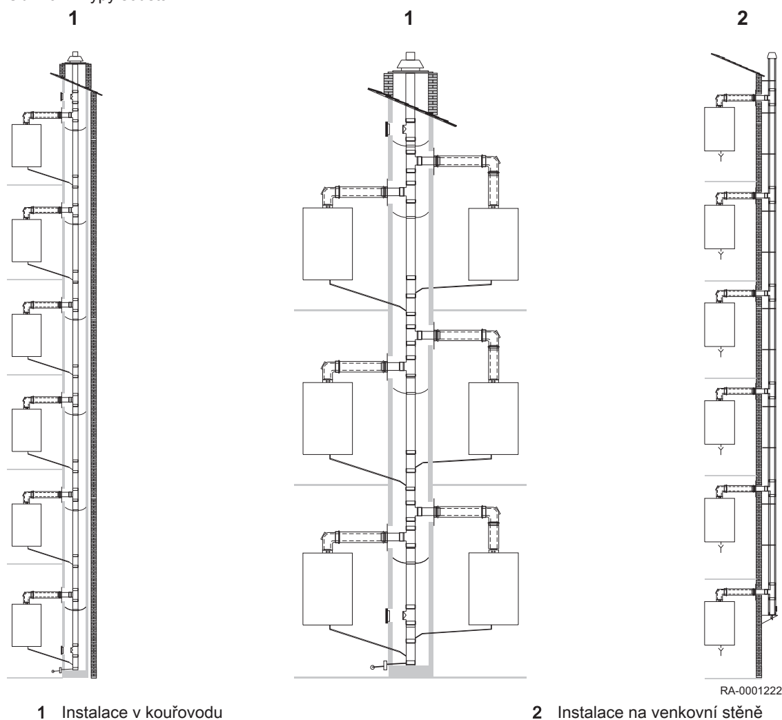
Obr.20 Typy soustav
