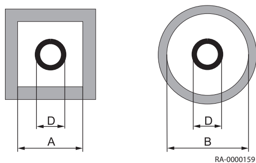
Obr.19 Minimální rozměry kouřovodu
