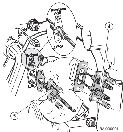
Obr.42 Demontáž zapalovací elektrody a ionizační sondy
