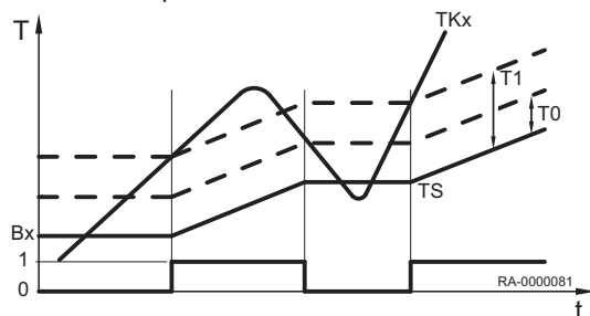
Obr.36 Naplňování zásobníku
