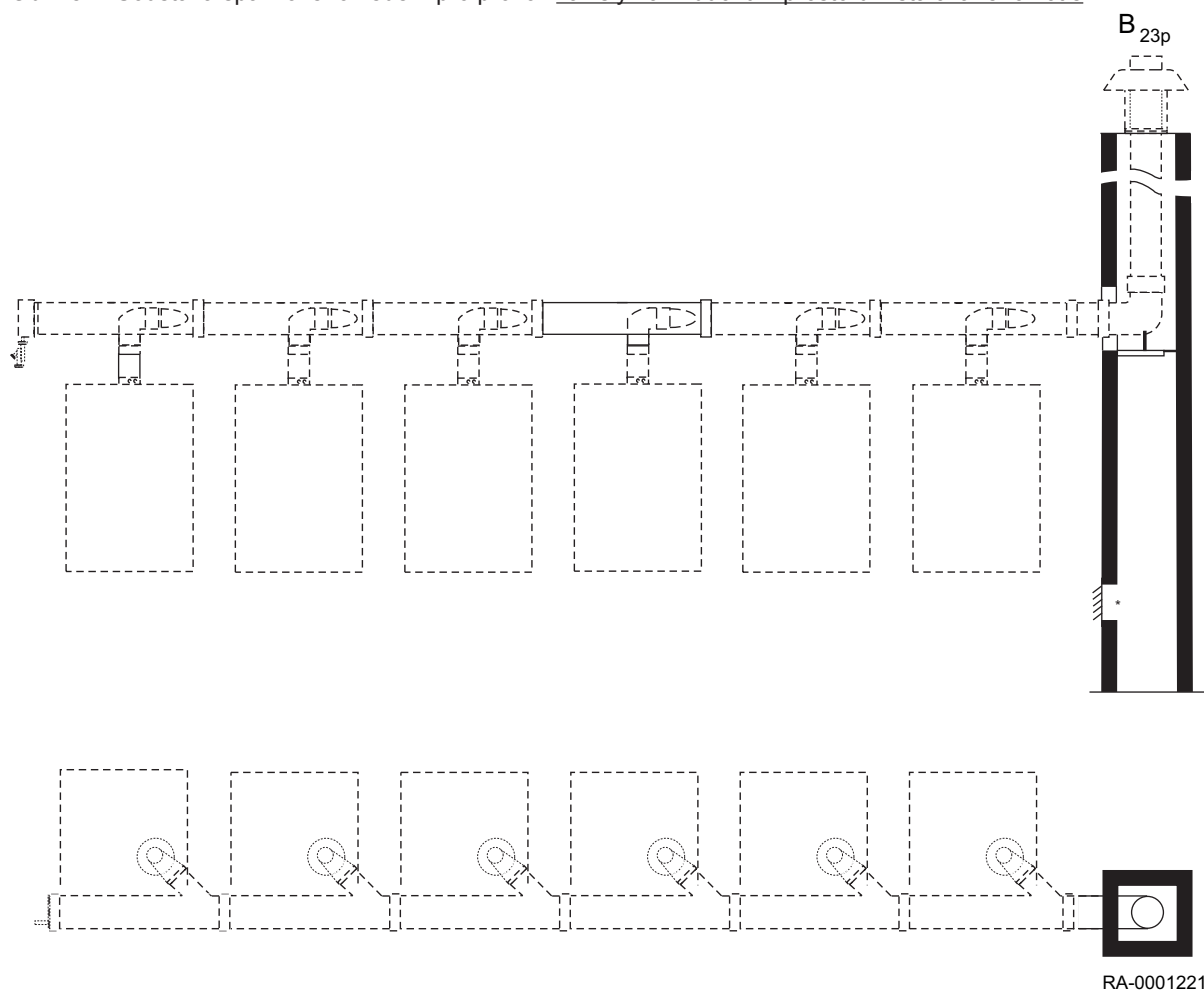
Obr.18 Soustava spalinového vedení pro provoz závislý na vzduchu z prostoru instalovaného kotle
