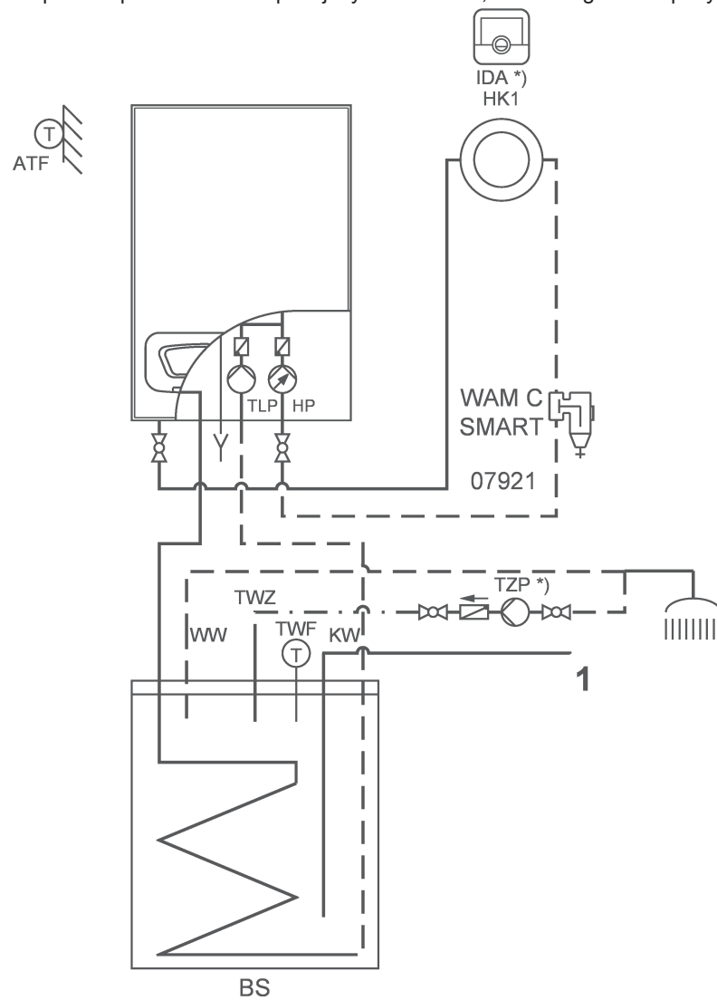
Obr.11 Příklad aplikace: Čerpadlo topného okruhu s pokojovým zařízením, včetně regulace teploty zásobníku
