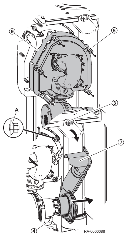
Obr.43 Demontáž hořáku
