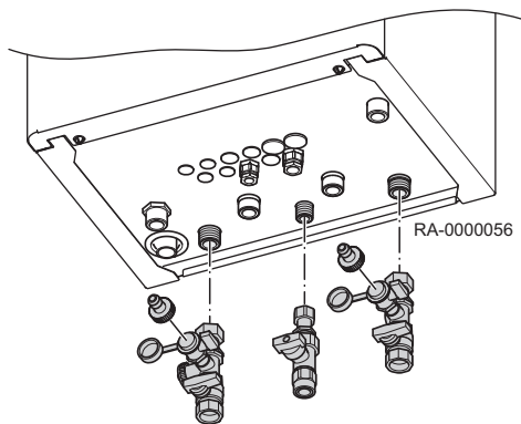
Obr.13 Instalace uzavíracích kohoutů
