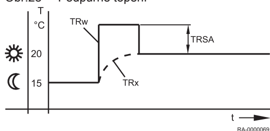
Obr.28 Podpůrné topení
