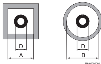
Obr.17 Minimální rozměry kouřovodu
