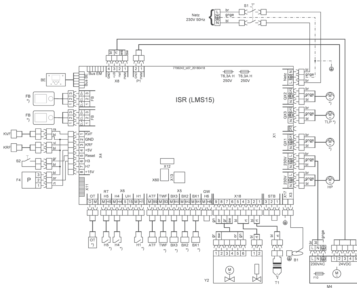
Obr.4 Schéma zapojení WGB EVO 15 – 28
