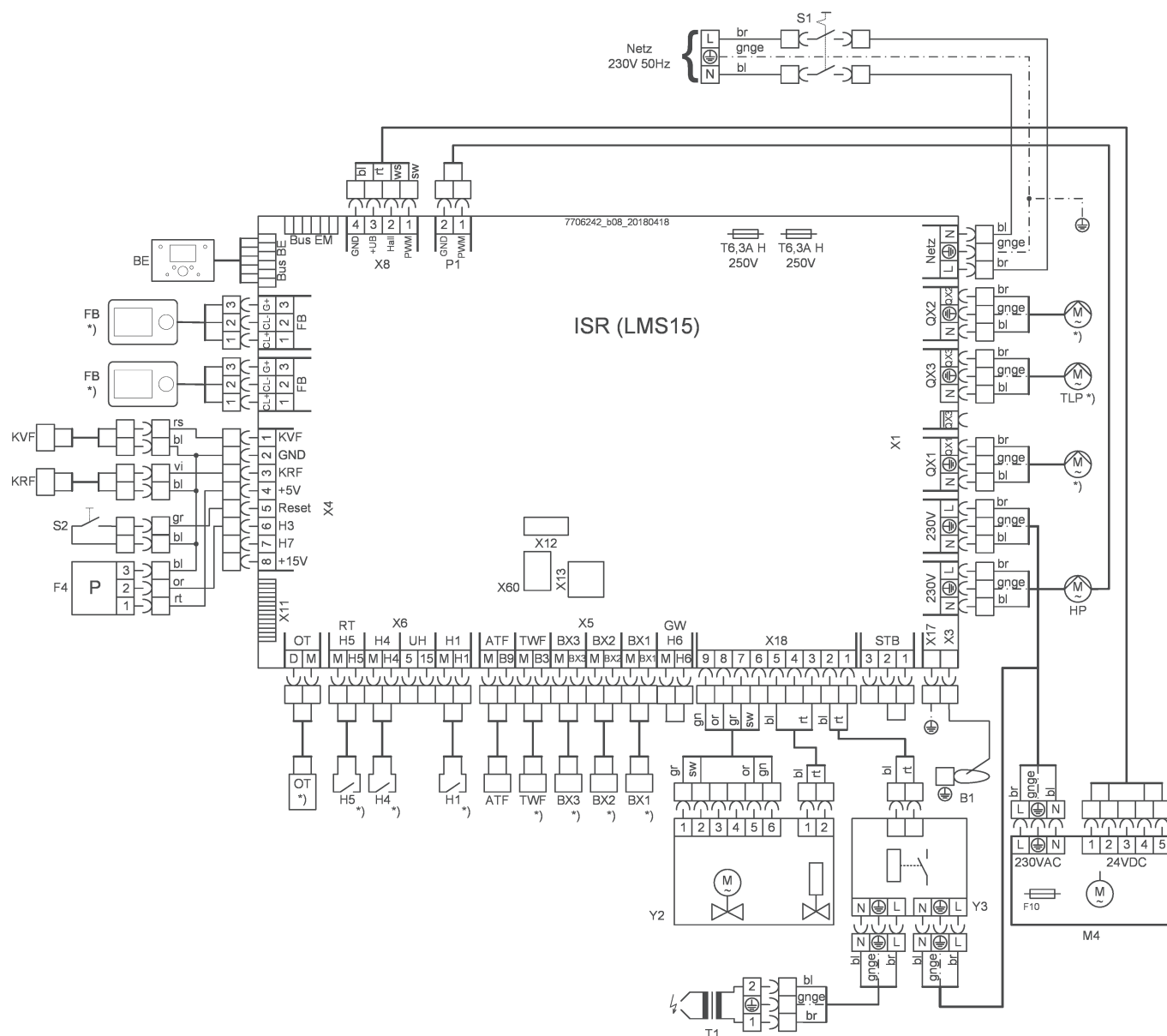
Obr.5 Schéma zapojení WGB EVO 38
