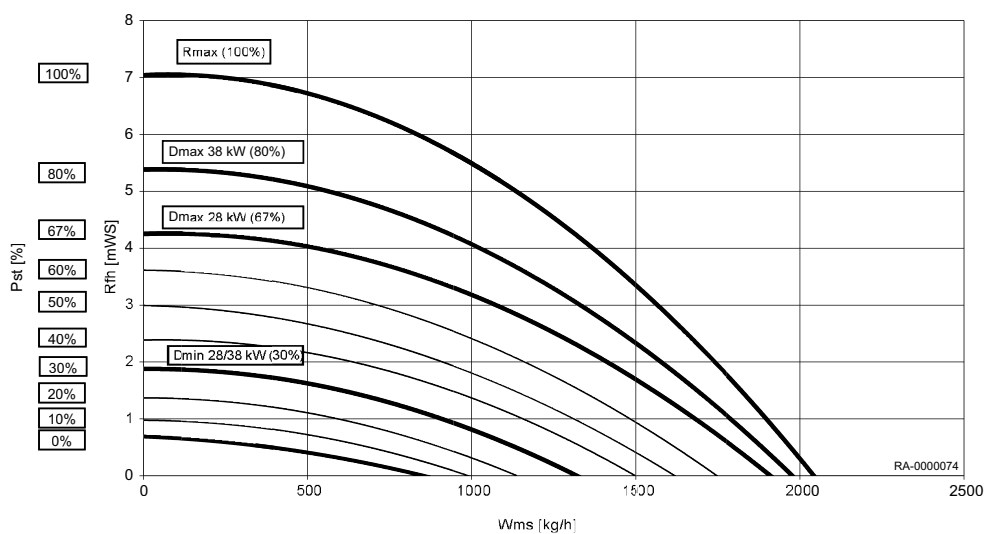
Obr.2 Celkový dynamický spád WGB EVO 28 – 38
