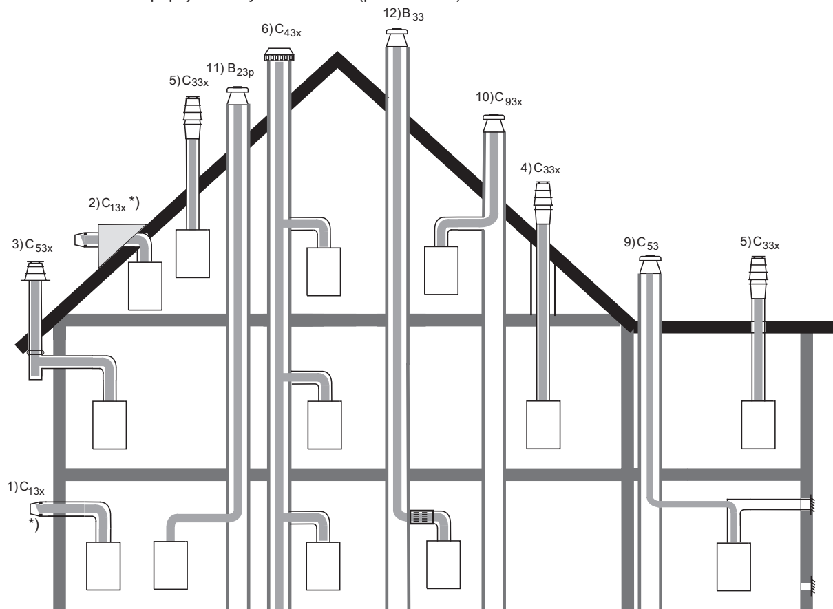
Obr.14 Možnosti připojení se systémem KAS (příslušenství)
