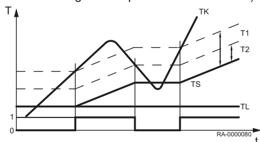
Obr.35 Regule napouštění /schematická)
