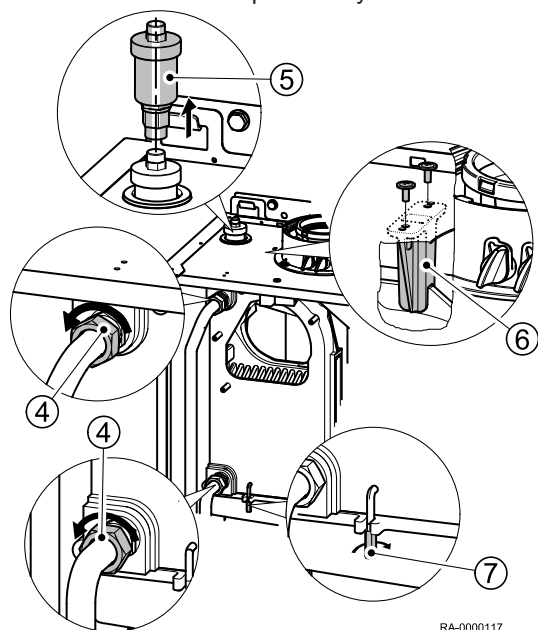
Obr.44 Demontáž tepelného výměníku
