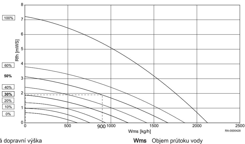
Obr.24 Příklad celkového dynamického počtu otáček
