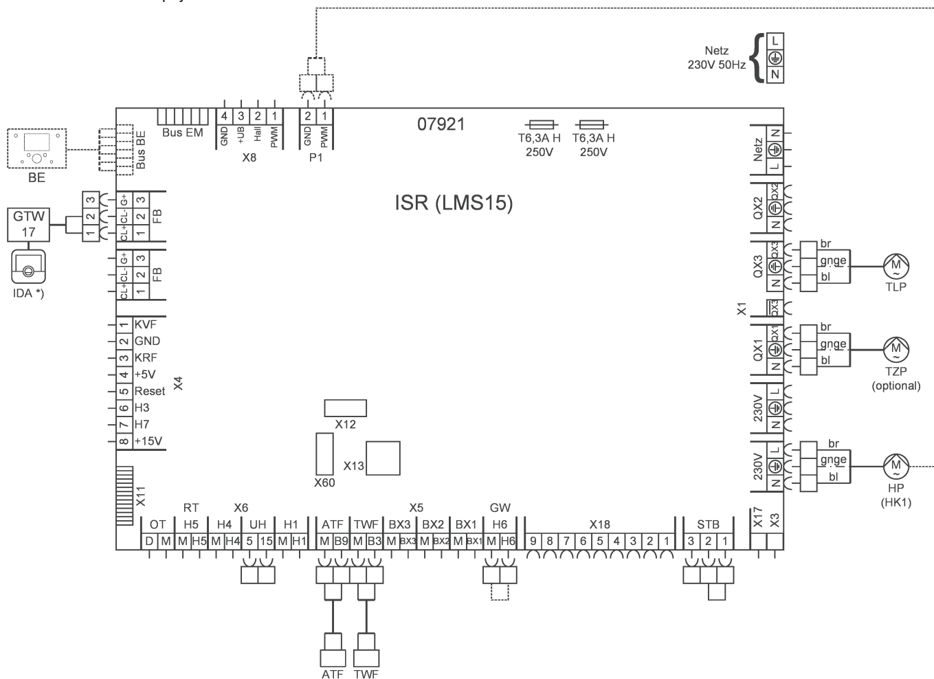
Obr.12 Schéma zapojení
