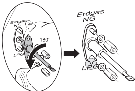
Obr.22 Změna na LPG
