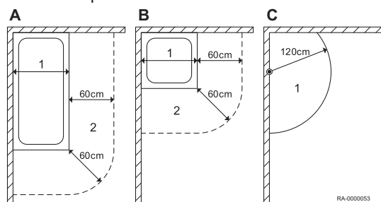
Obr.10 Volné prostory v koupelně a ve sprše
