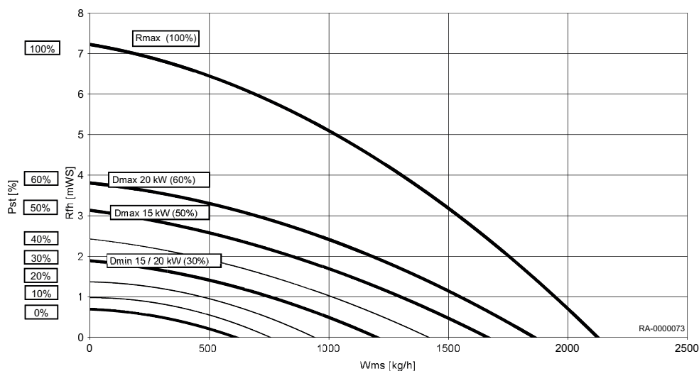
Obr.1 Celkový dynamický spád WGB EVO 15 – 20
