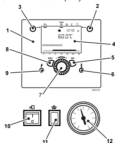
Obr.7 Provozní prvky
