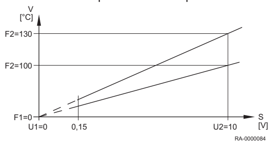
Obr.39 Příklad požadavku na teplo 10 V
