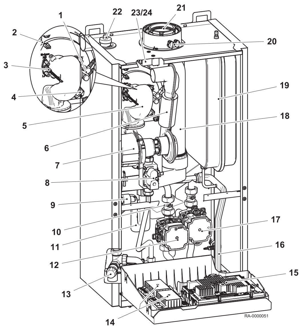
Obr.6 Náhled na kotel WGB EVO (zobrazení bez přední stěny a krytu regulační jednotky)
