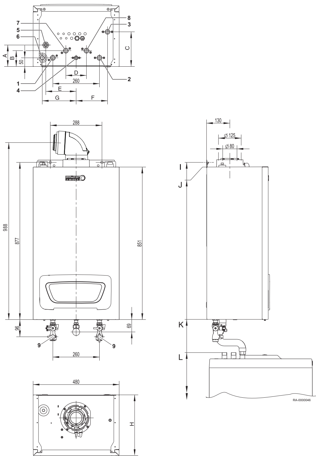
Obr.3 Rozměry a připojení WGB EVO
